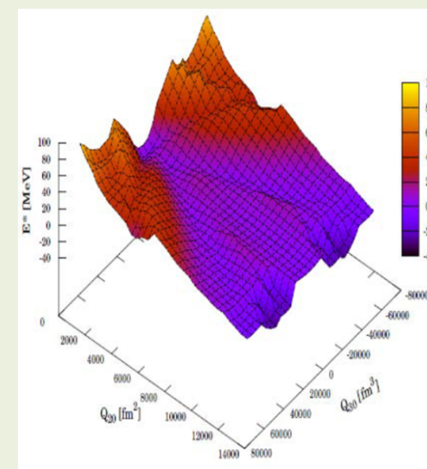
^{236}\text{U} の Q_{20} と Q_{30} に関するエネルギー面
