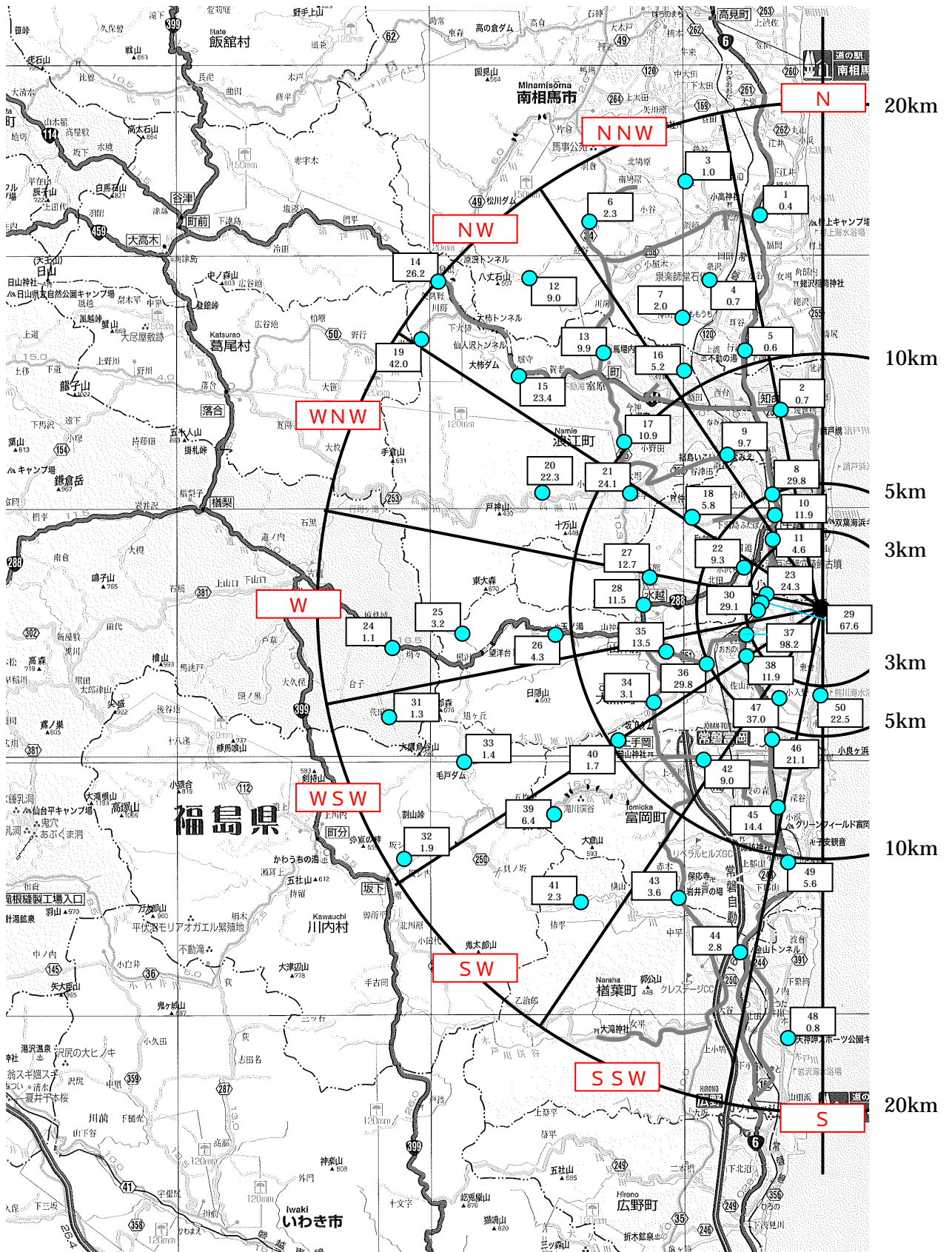
福島第一核电站 20km 范围内空中核辐射含量检测结果 ( 测量日 : 2011 年 5 月 27 日 )
