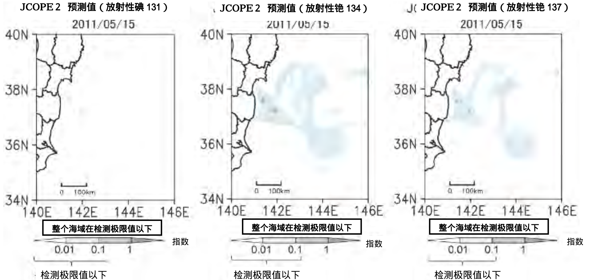
【图3 - 1】JCOPE2 模拟的放射性物质含量分布 - 5月15日 - (根据5月3日为止的数据所做的模拟)
