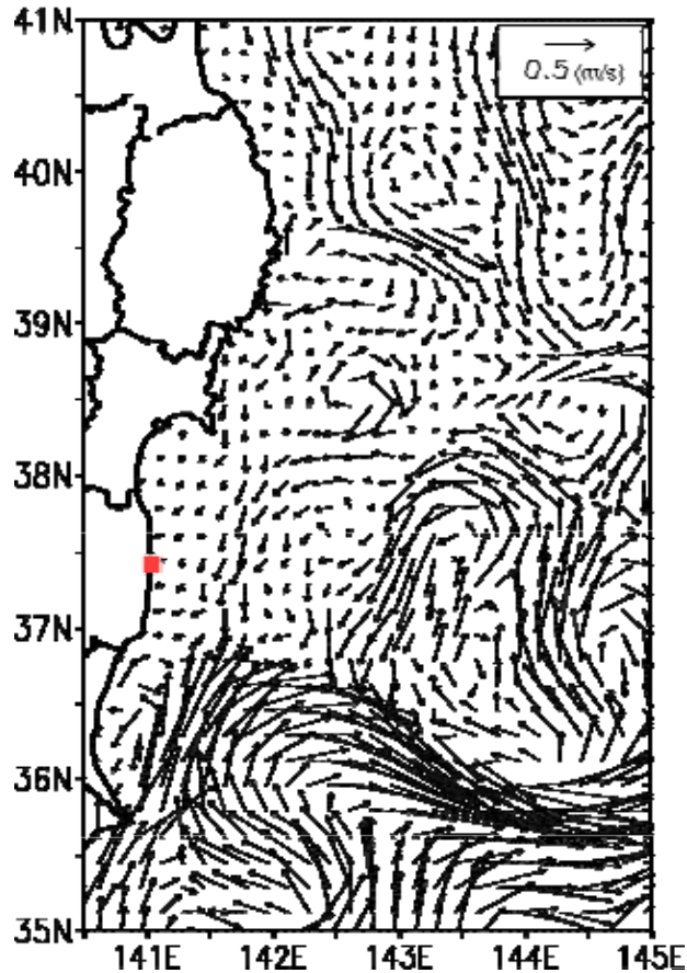
【图 2】JCOPE2 的速度分布 (5月3日)
