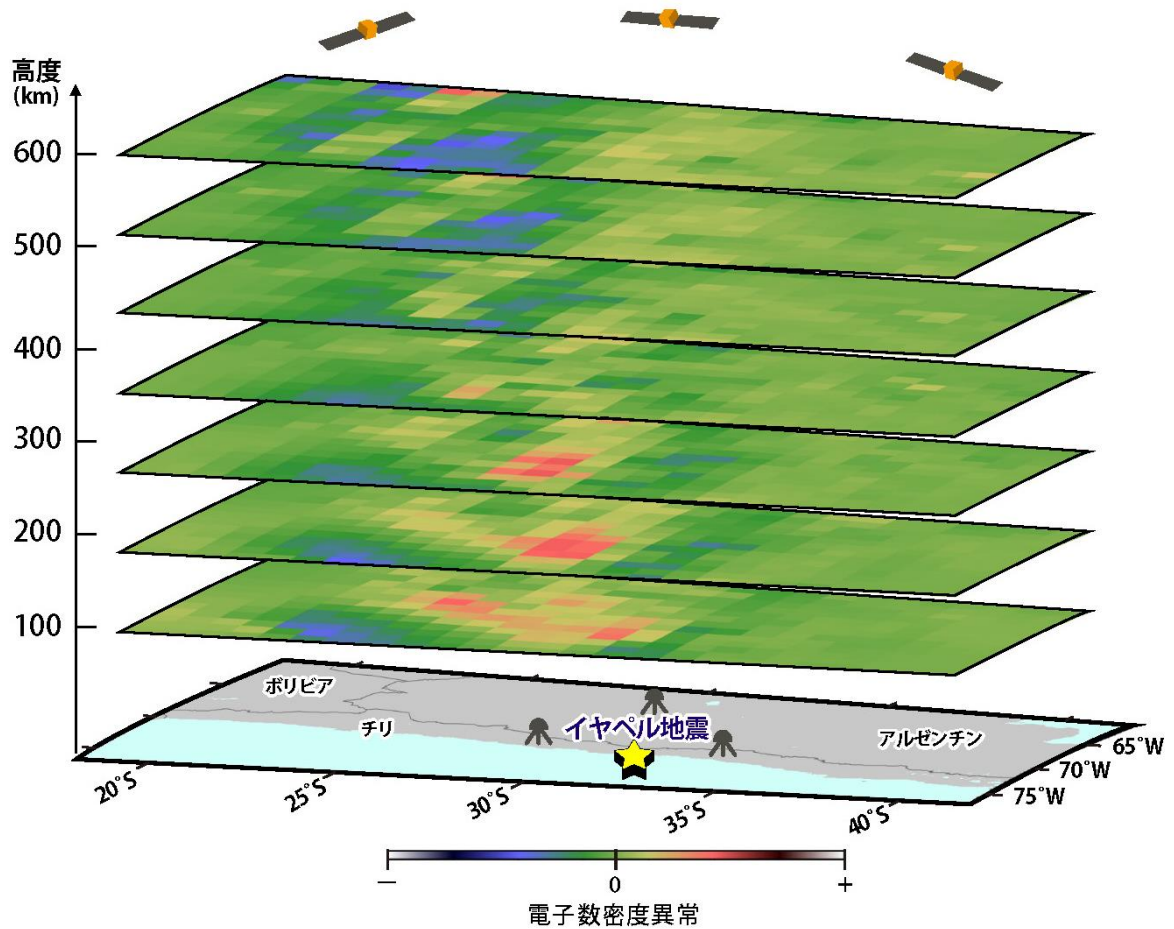
図1 1 巨大地震に先行する電離層の電子数密度変化
