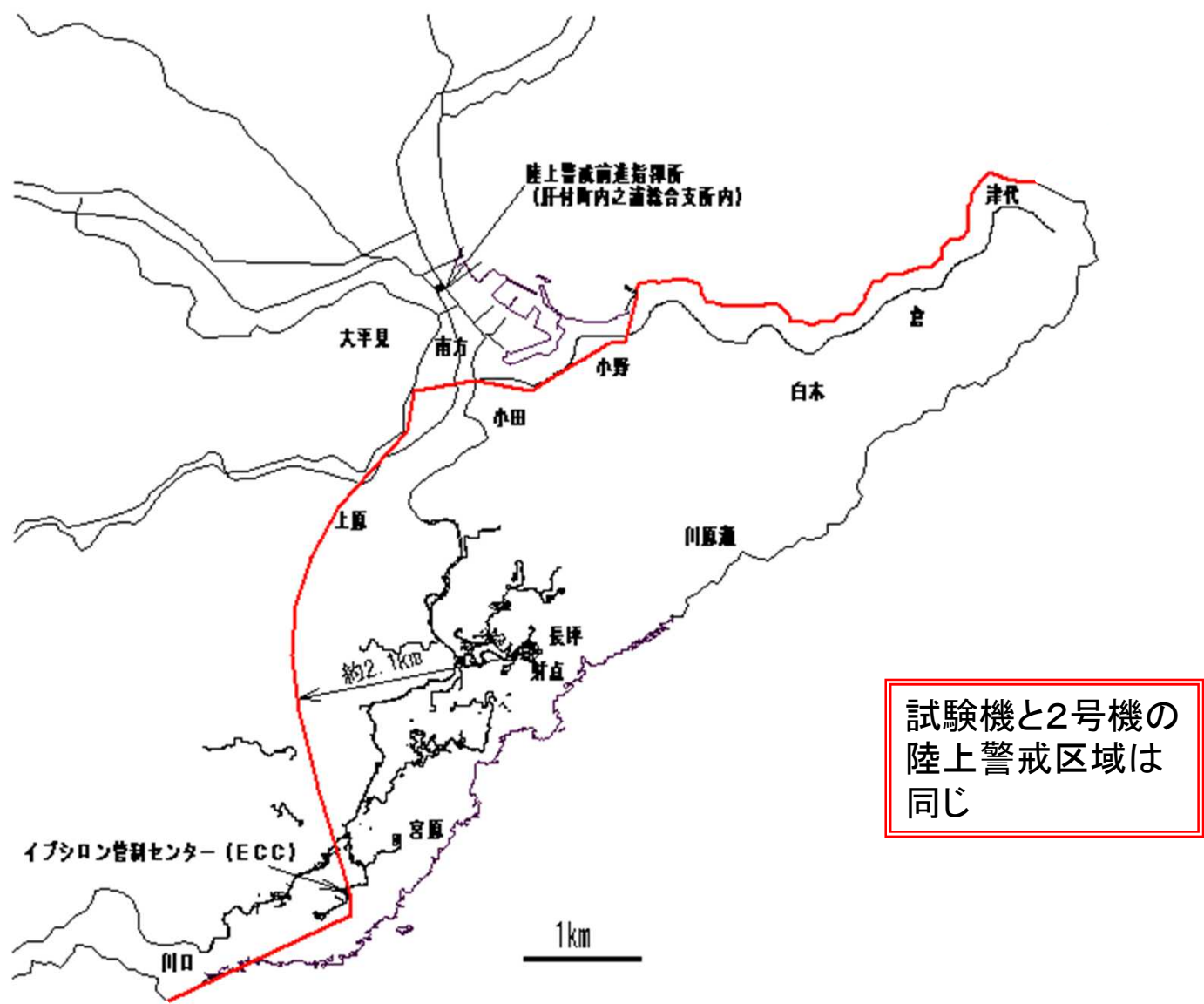
図3: 陸上警戒区域
