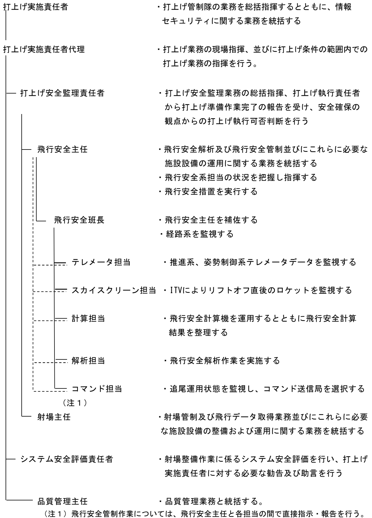
図9 飛行安全関連組織
