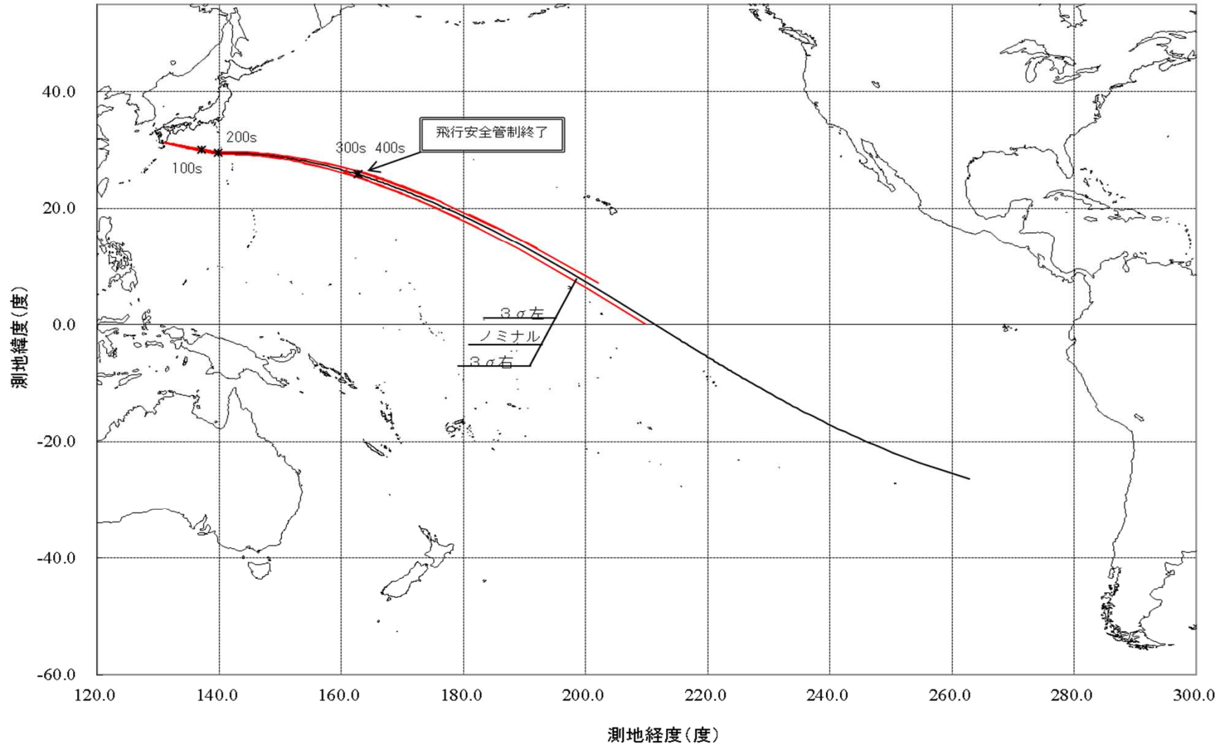
図9:ロケットの落下予測点(注)軌跡と3σ分散範囲
