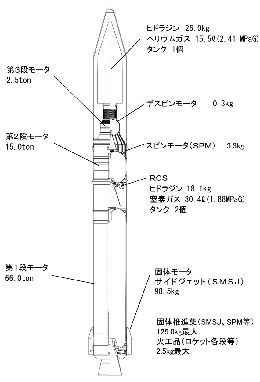
図1:ロケット等搭載用保安物
