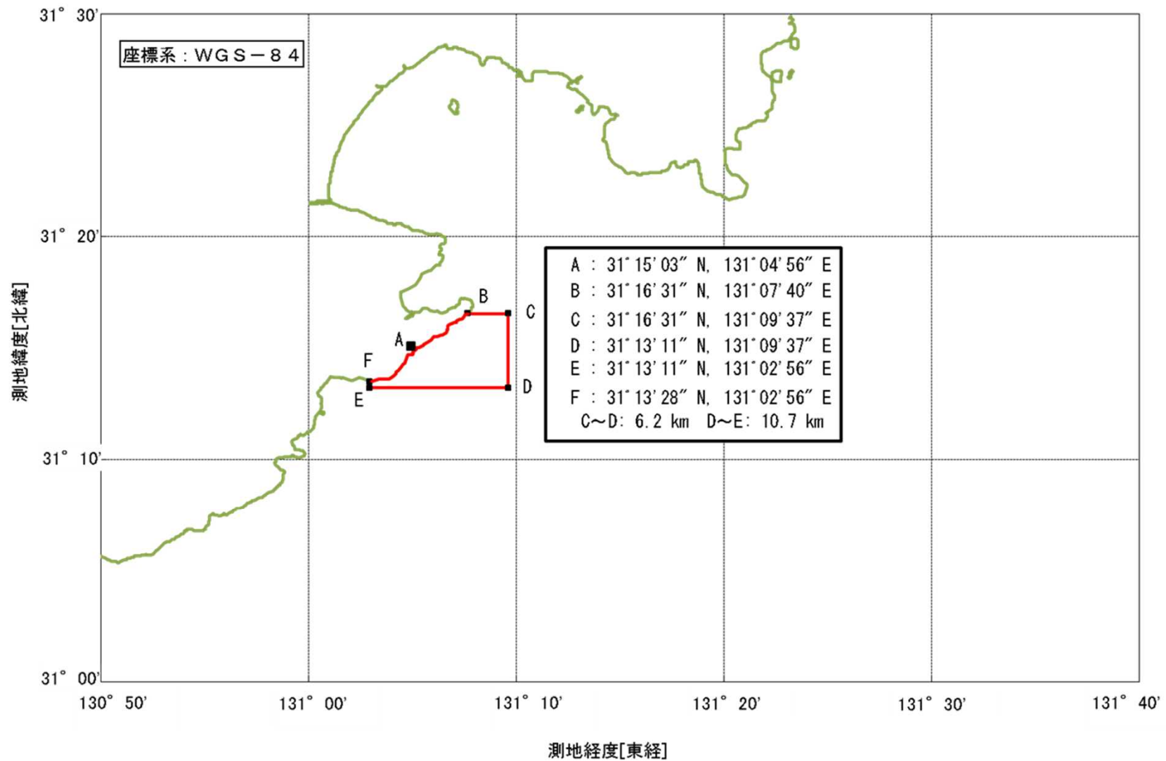
図5-1:水路通報のための海上警戒区域
