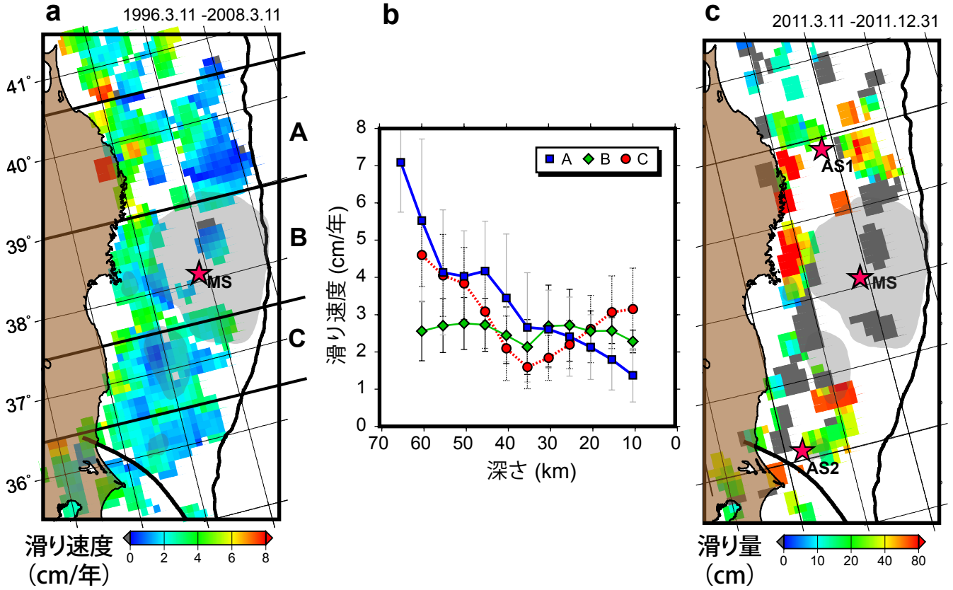
東北地方太平洋沖地震 発生前の滑り速度
