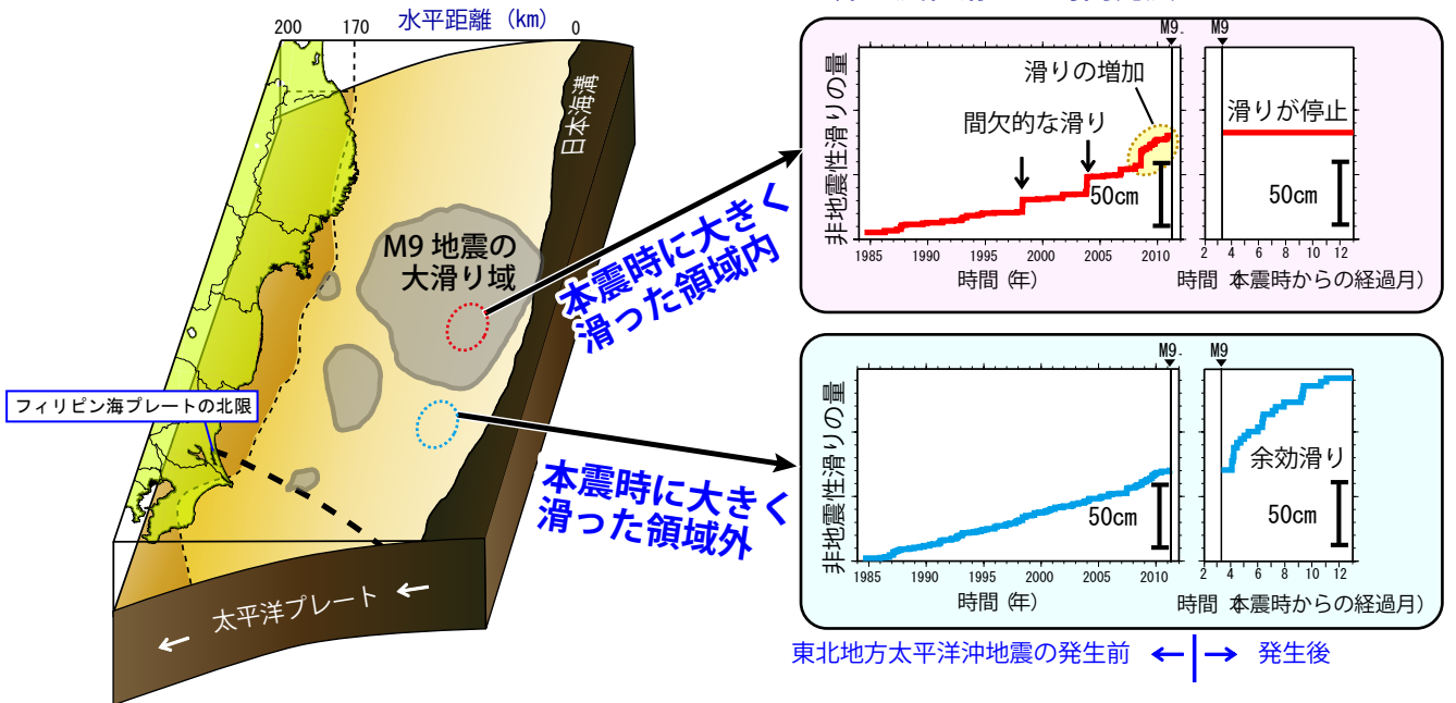
図15 (東北地方太平洋沖地震の前の非地震性滑り) 上図：(a) 東北地方太平洋沖地震発生前のプレート境界の非地震性滑りの平均滑り速度分布, (b) A～Cの3領域において平均した滑り速度の深さ変化を示す。(c) 本震発生後9か月間の非地震性滑りの滑り量分布を表す。下図：本震発生前後の非地震性滑りの時空間発展の概念図。
