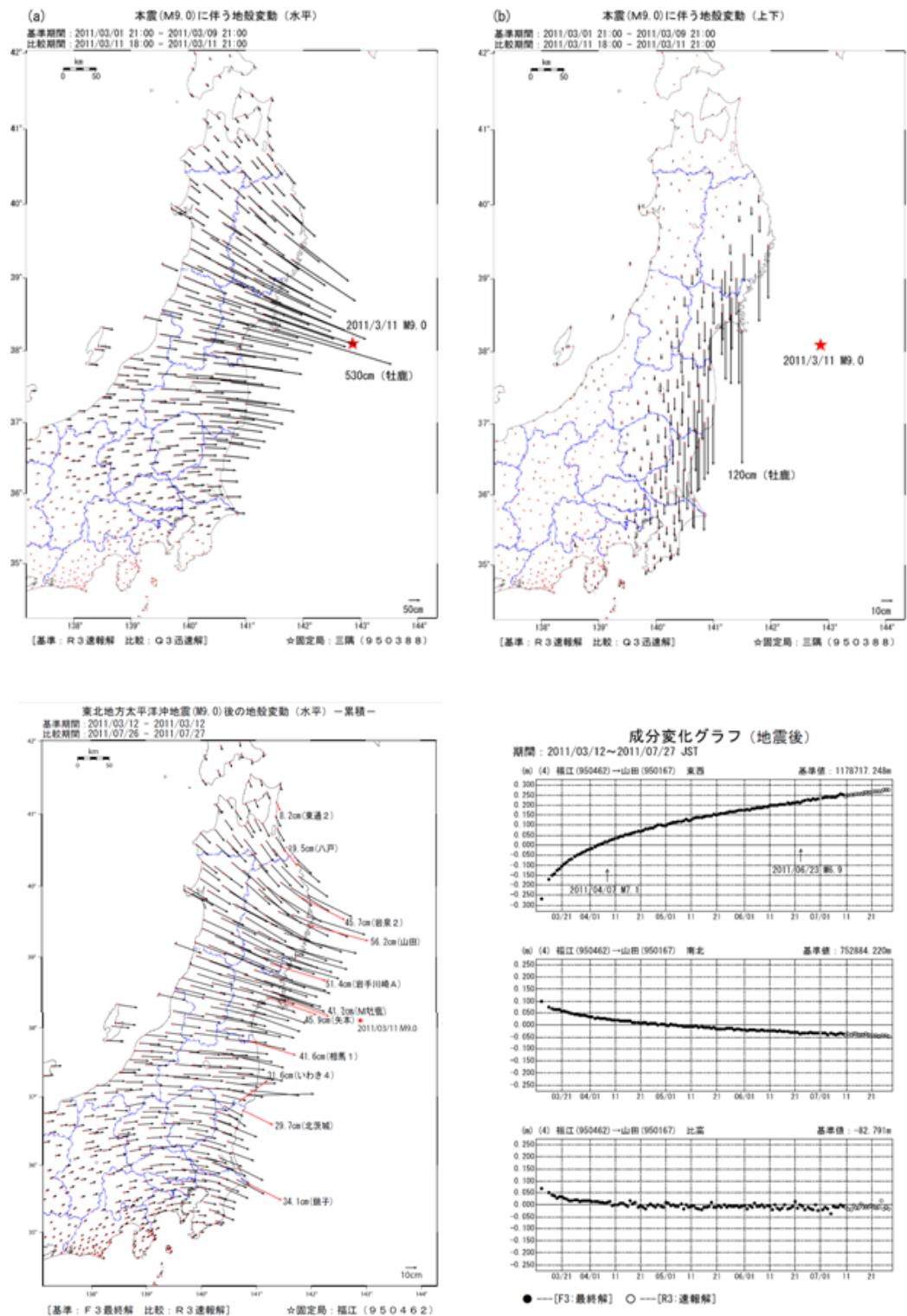
図2 東北地方太平洋沖地震に伴う地殻変動量(上段(左):水平成分,(右):上下成分),及び地震後(3~7月)の余効変動量(下段(左):水平成分,(右):電子基準点「山田」時系列)(国土地理院[課題番号:6001])
