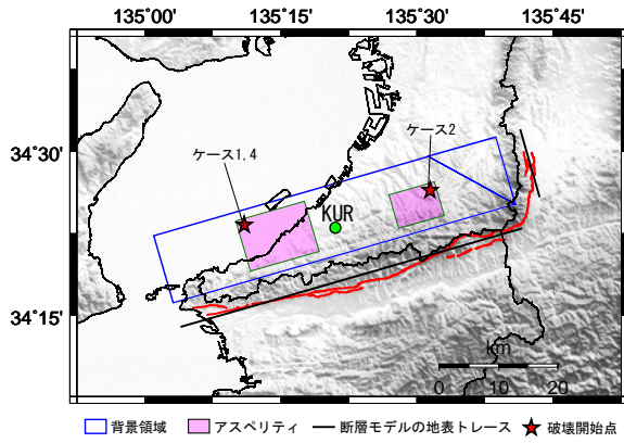
(a) 断層配置図 (ケース 1,2,4)
