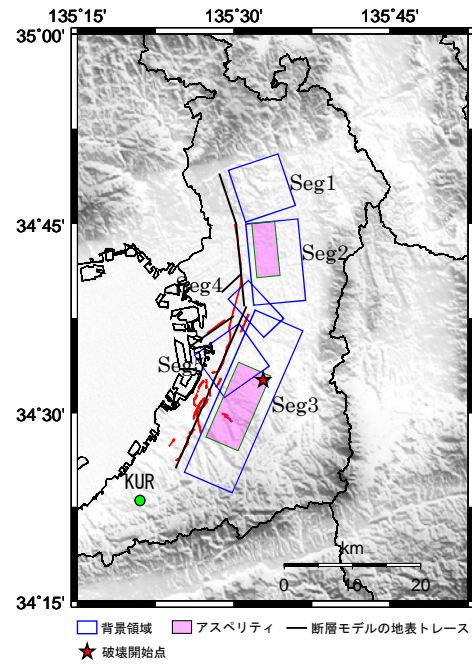
(b) 断層配置図 (ケース 2)
