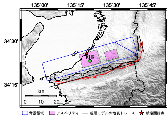
(b) 断層配置図 (ケース 3)
