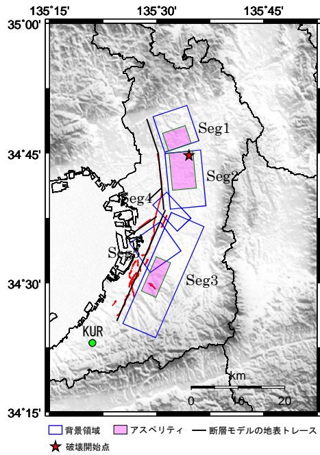
(a) 断層配置図 (ケース 1,3)
