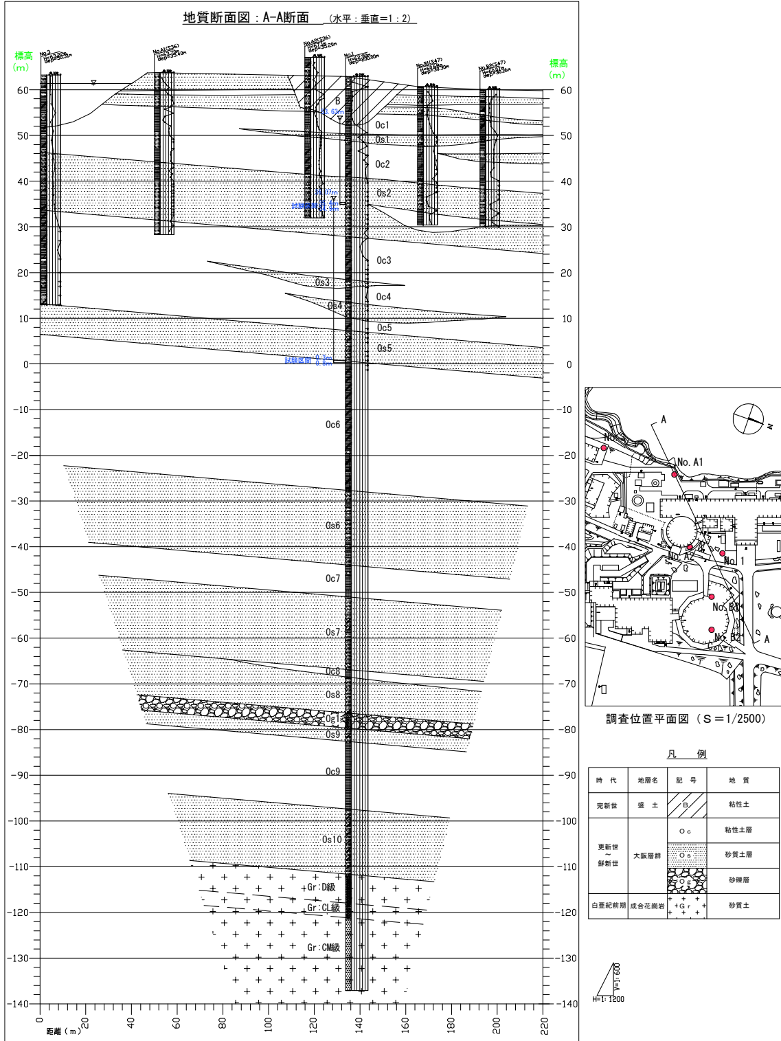
図3-2-1 地質断面図 (SH=1/1,200, SV=1/600)
