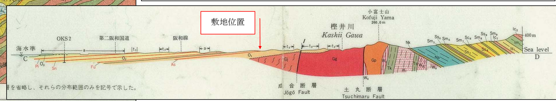
第 3.3.2-2 図 調査地周辺の地質図 5 万分の 1 地質図副「岸和田地域の地質」地質調査所 (1986) ①に加筆
