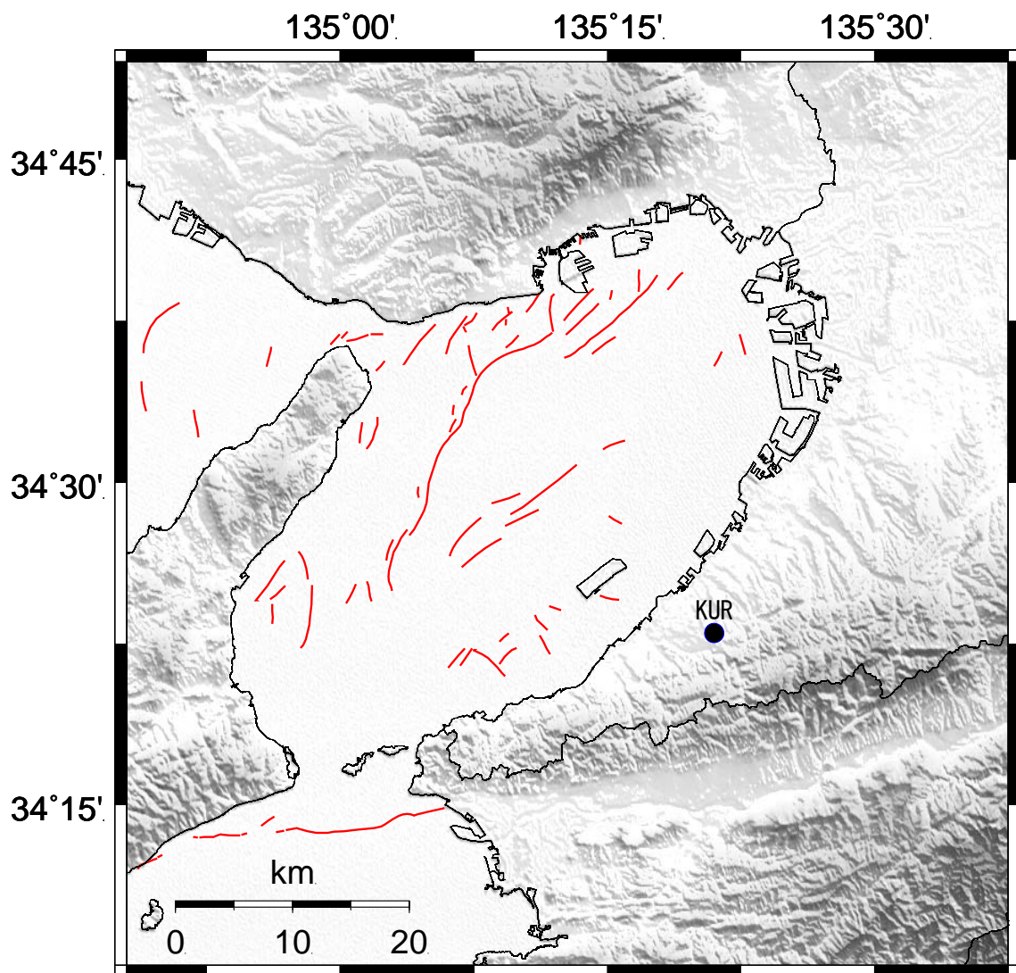
第 3.2.2-19 図 大阪湾と周辺の構造図 (海上保安庁水路部, 1995 (75) )
