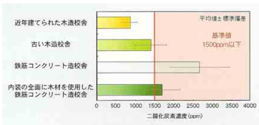
図2 冬期の教室内の平均二酸化炭素濃度 （木質内装で快適な生活を・文部科学省 都市エリア産学官連携促進事業（米代川流域エリア）2009）
