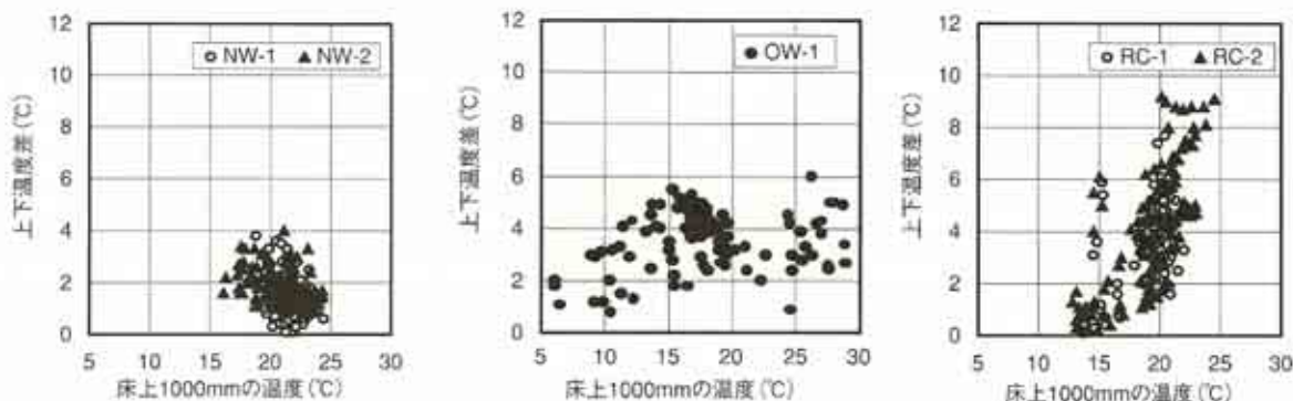
図1 校舎の構造別の教室内の温度と上下温度差の分布 （木村彰孝、小林大介、飯島泰男：教室内の環境が子どもにもたらす影響に関する研究 その2 能代市内小学校における冬期の温熱環境と子どもの評価・日本建築学会大会学術講演梗概集（関東）2009）
