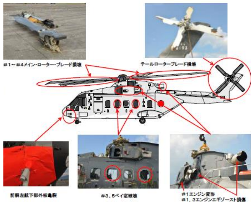
機体の損傷状況(左側)
