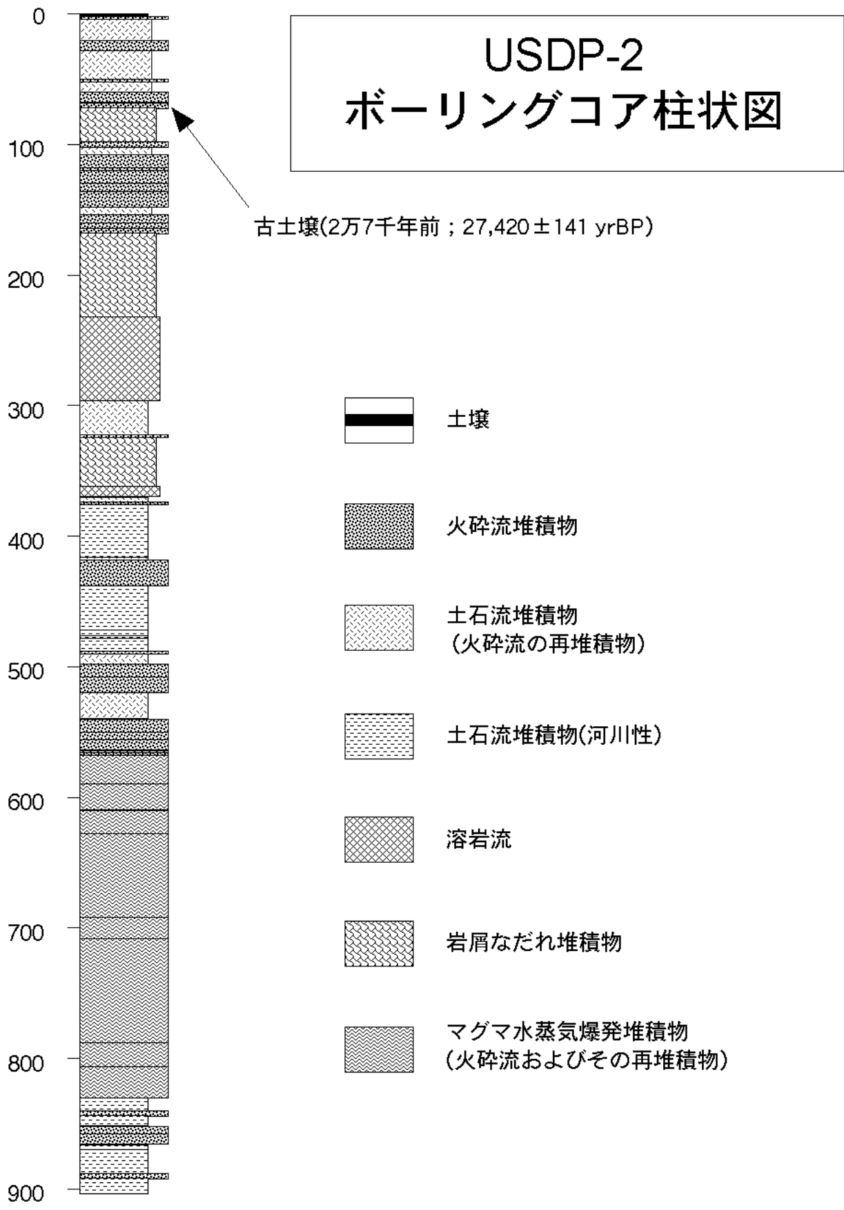
図1 H12年度掘削柱状図
