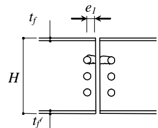
図 3.5.6 端抜け破断
