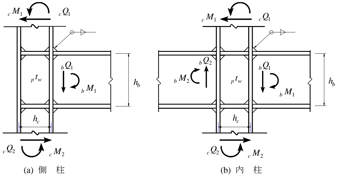
図 3.4.3 柱梁接合部
