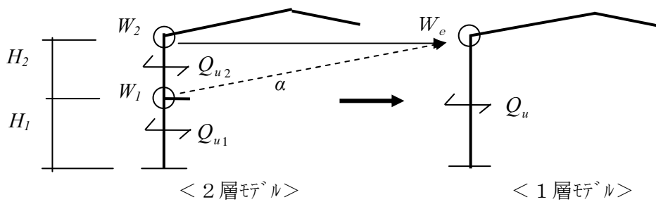
図 4.3.2 高さ比置換図
