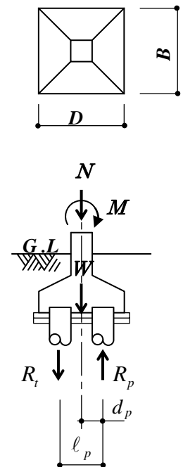
図 3.9.2 くい基礎の転倒抵抗モーメント
