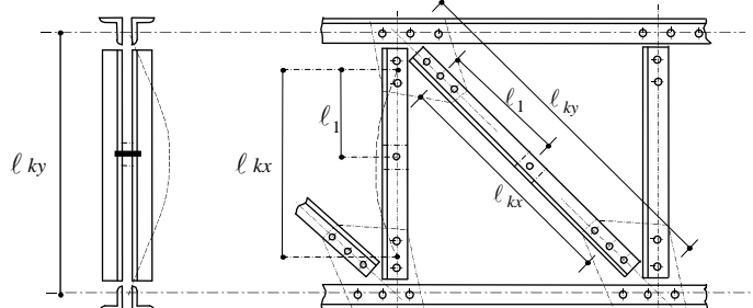
図 3.2.5 ラチス材の座屈長さ
