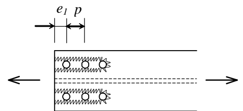
図 3.5.2 端抜け破断
