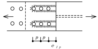
図 3.5.5 中抜け破断
