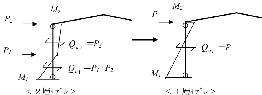
図 4.3.4 等価応力図
