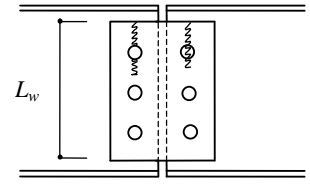
図 3.5.8 端抜け破断
