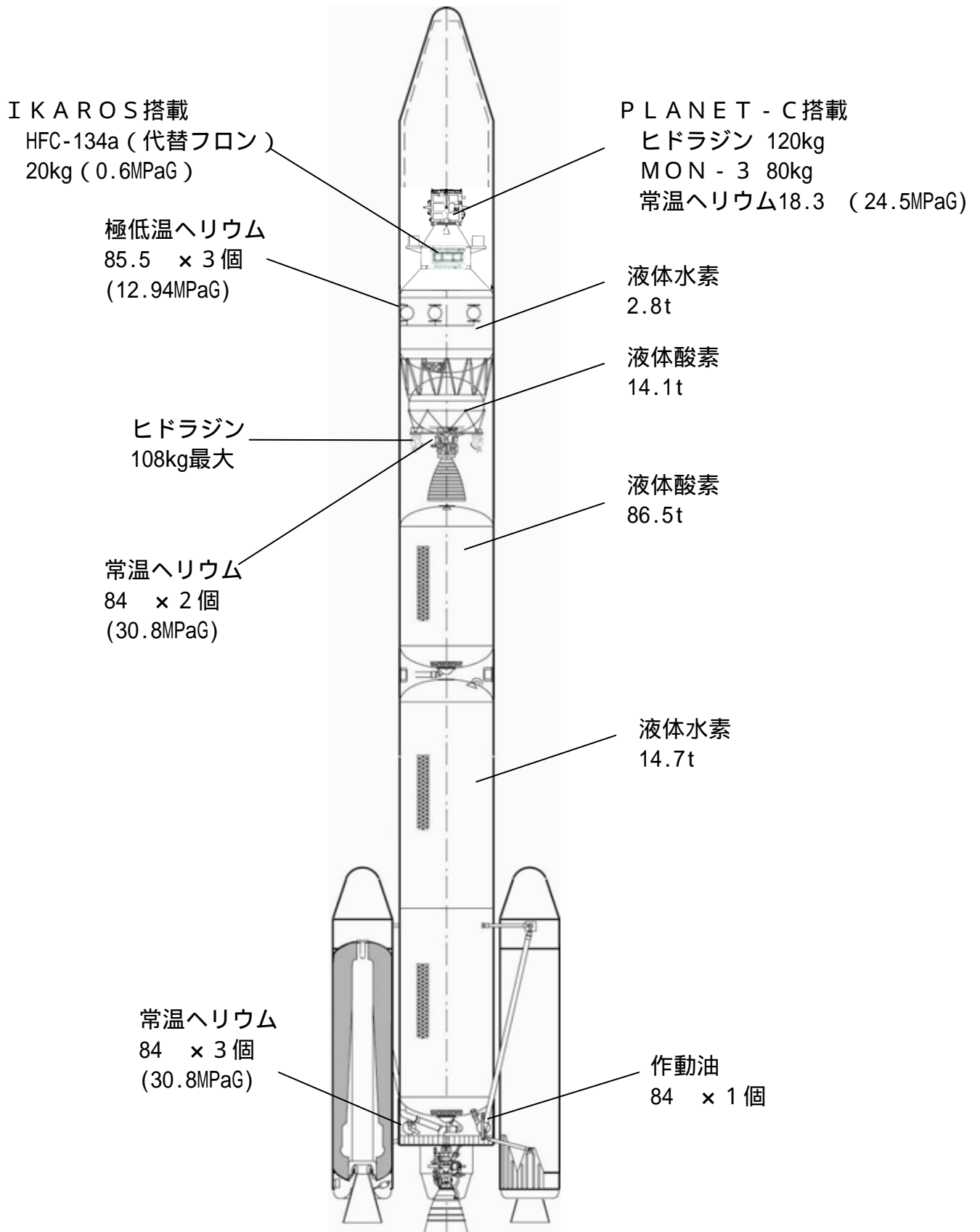
図 - 1 H - A ロケット搭載保安物概要 ( 高圧ガス、危険物等 )
