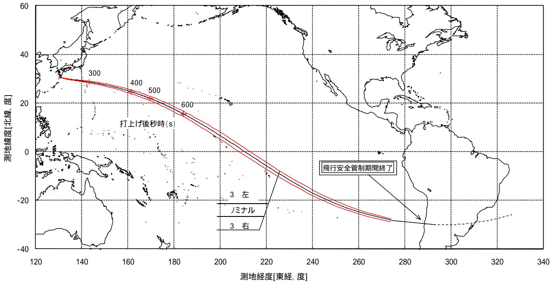
図 - 8 ロケットの落下予測点 (注) 軌跡と3 分散範囲 (注) 落下予測点：ある時点でロケットの飛行を中断した場合の、ロケットあるいは生成破片の落下予測点
