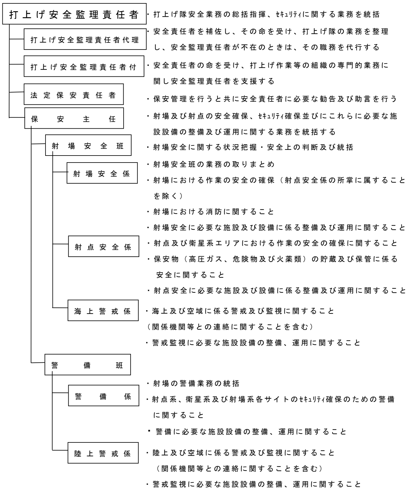
図－１２ 地上安全組織及び業務
