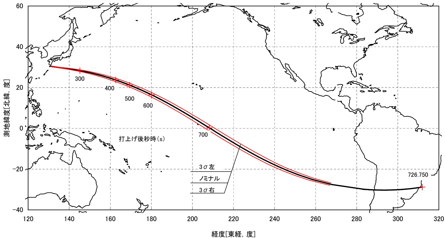
図-8 ロケットの落下予測点軌跡と3σ分散範囲
