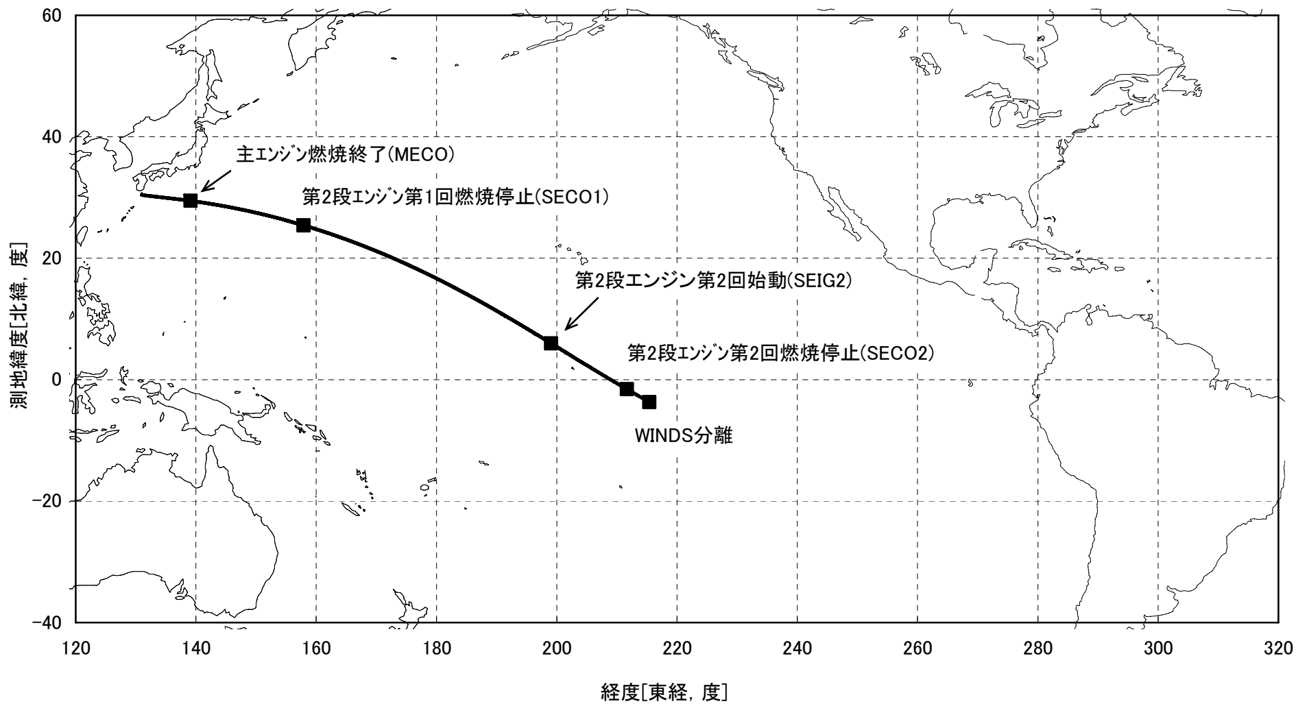
図-6 H-II A ロケット 14 号機の飛行経路
