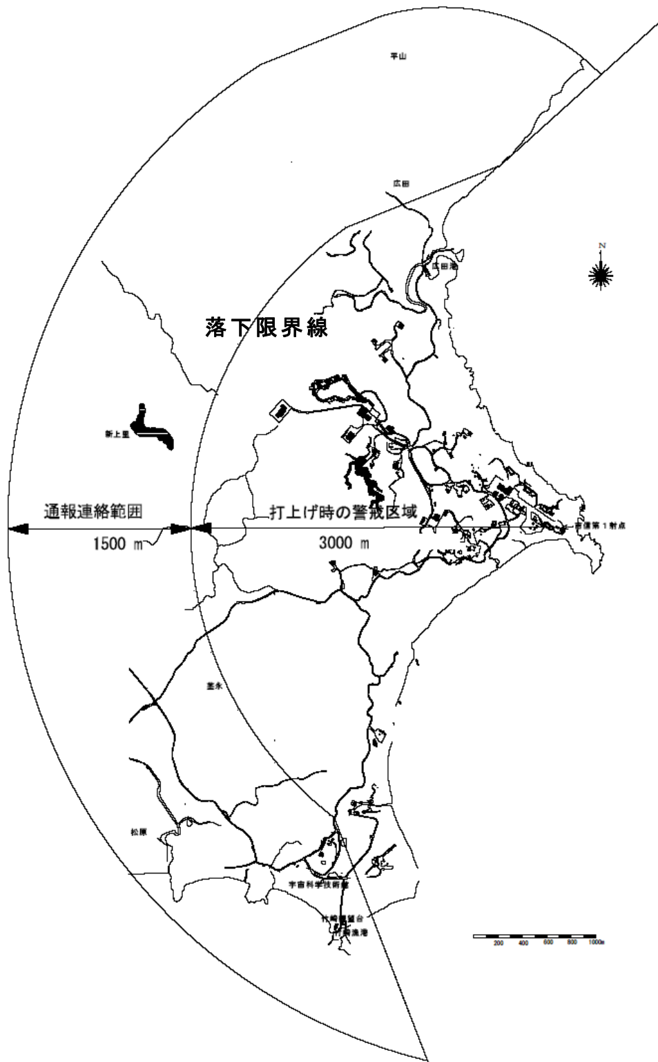
図一 4 ガス拡散範囲に係る通報連絡範囲及び落下限界線
