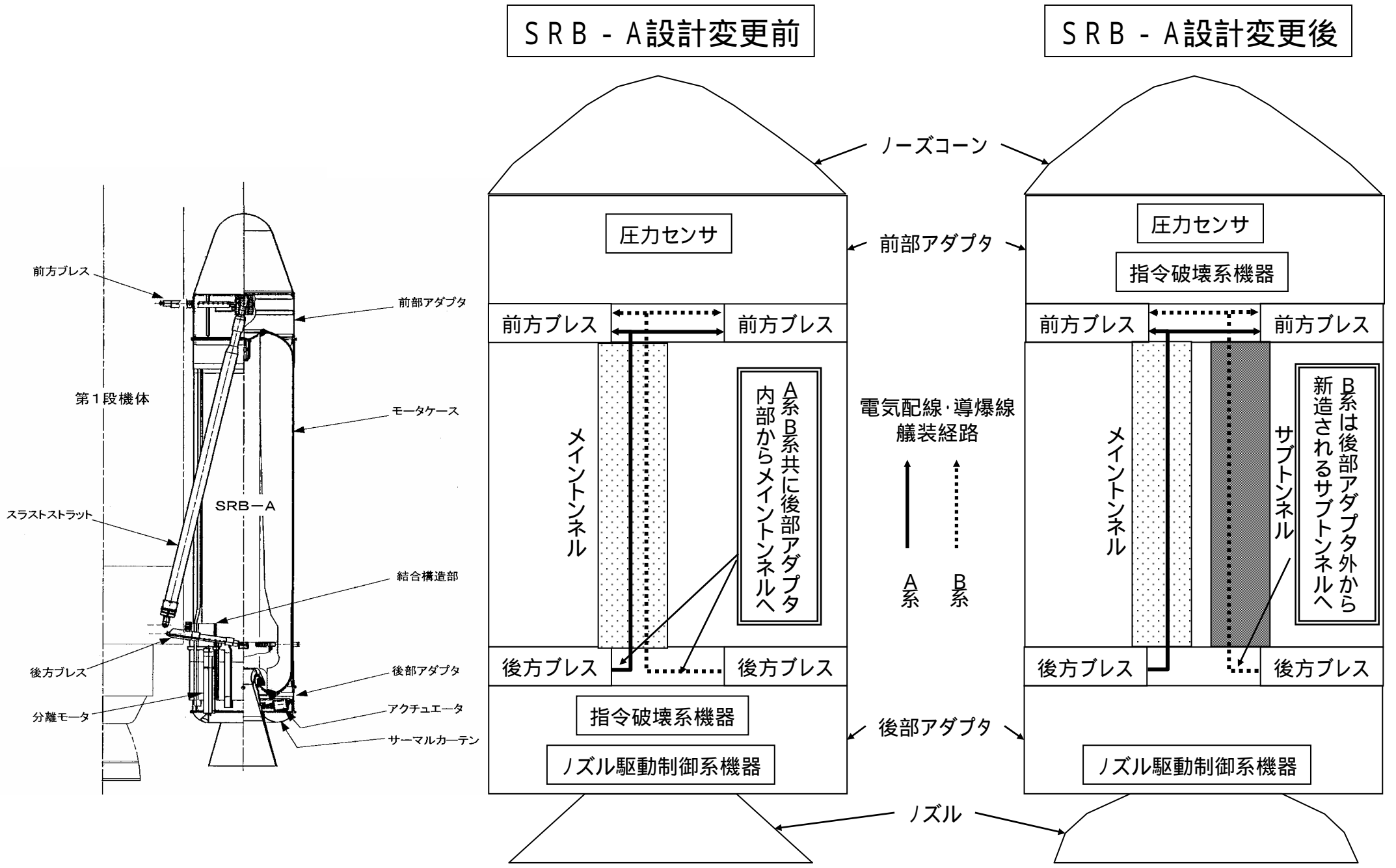
図2 導爆線及び電気配線等の艦装の設計変更案概要
