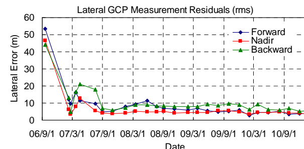
画素地表位置決定精度の長期トレンド * (経度方向)
