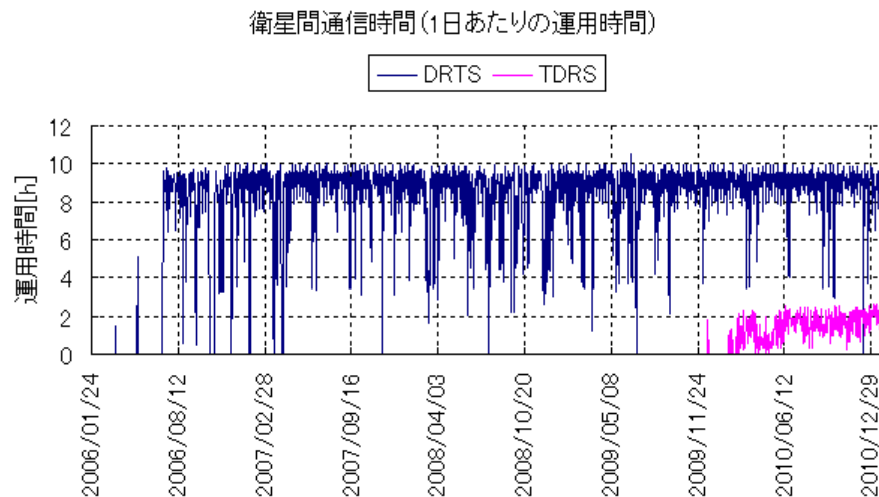
衛星間通信アンテナ(DRC)運用時間 <DRTS 8.8h/13.4回/日、TDRS 1.6h/3.9回/日(半年間の平均)>
