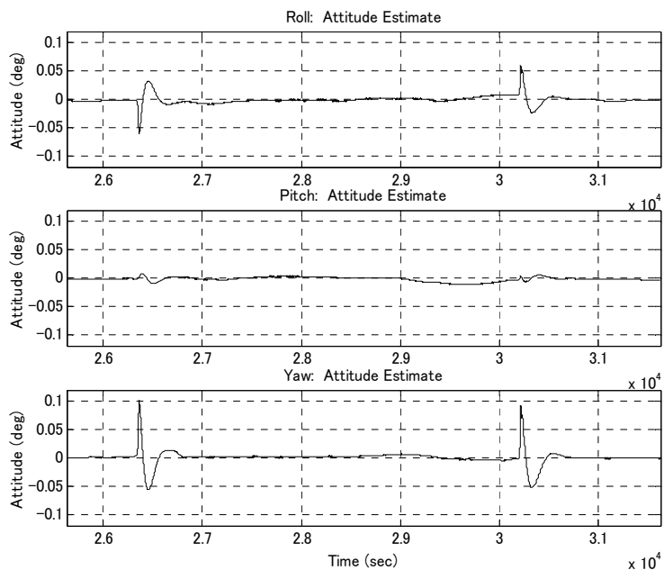
姿勢制御精度 (周回誤差プロファイル)
