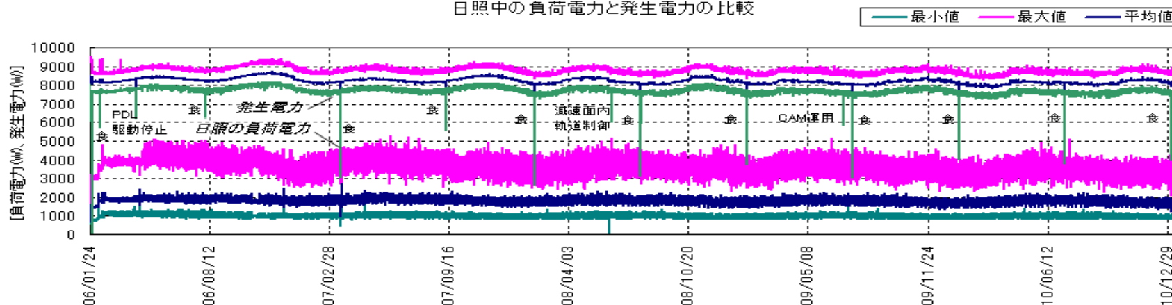
発生電力 8Kw(上段グラフ)。日食による発生電力の低下(年2回)
