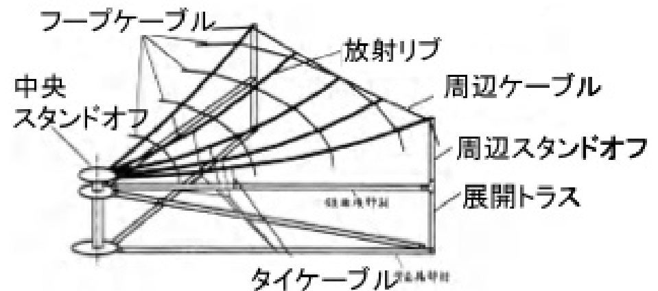
放射リブ／フープケーブル方式
