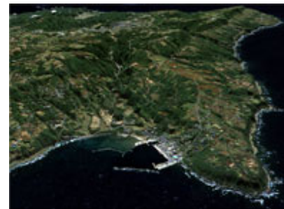
標高データを利用した 種子島鳥瞰図
