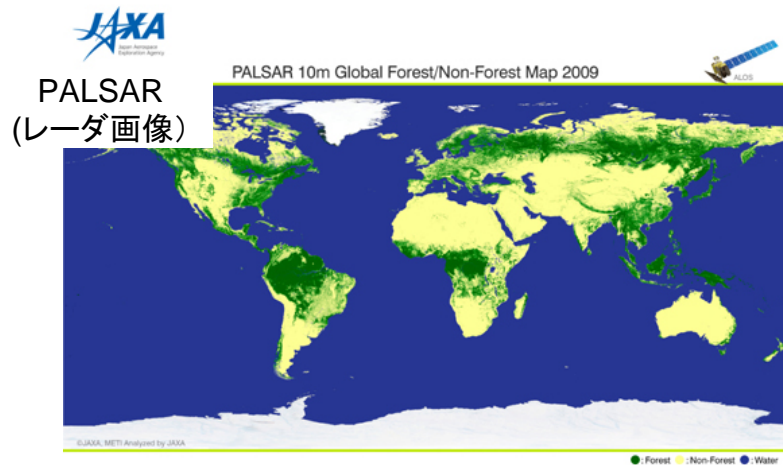
全球森林・非森林分類図(平成21年分)
