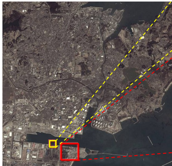
ALOS-3シミュレーション画像(分解能0.8m)
