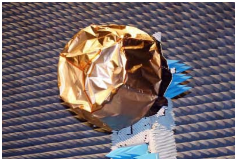
19素子ヘリカルアレイアンテナ
