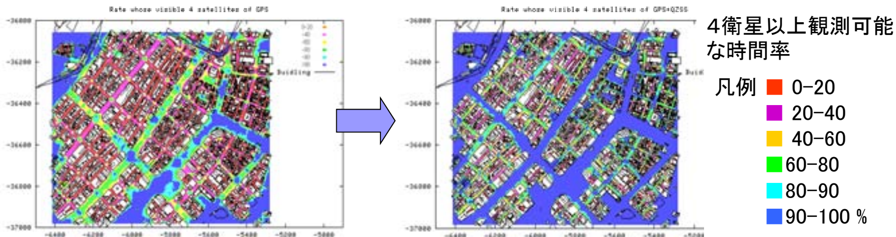
都市部でのアベイラビリティ増大例(東京銀座地区3Dシミュレーション)
