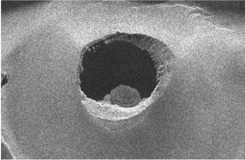
図2 噴火中の浅間山山頂火口の合成開口レーダー画像（2004年9月16日撮影。国土地理院による）。航空機搭載型合成開口レーダーによって北側から撮影された（画面上が北）。火口底に渦巻き模様の表面構造を持つ饅頭状溶岩塊が認められる。
