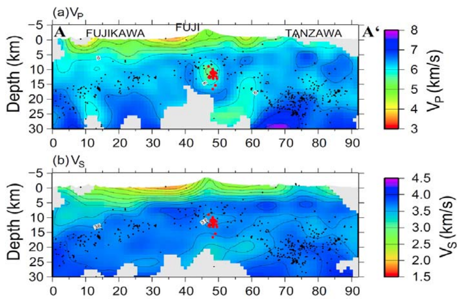
図2 自然地震により求められた地震波トモグラフィ。南西-北東断面。山頂直下10~15 km 付近に分布する赤点は、深部低周波地震の震源位置で、低速度領域の位置と一致している。また、山頂直下20km以深に別の低速度領域の存在が示唆される。
