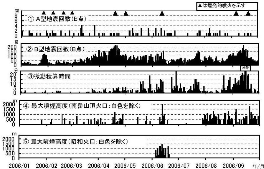
図2 桜島の火山活動の経過（2006年1月1日～9月30日）
