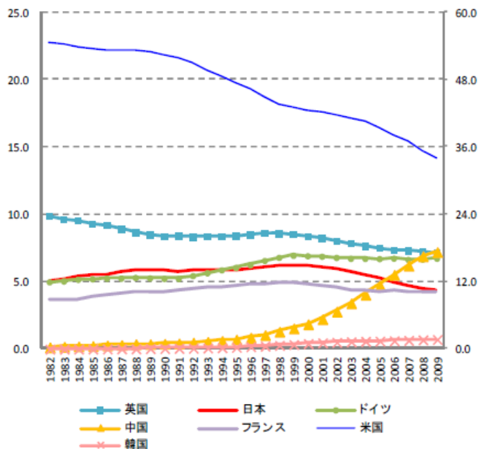
全分野でのTop10%補正論文数(3年移動平均%) (分数カウント、米国は右軸)
