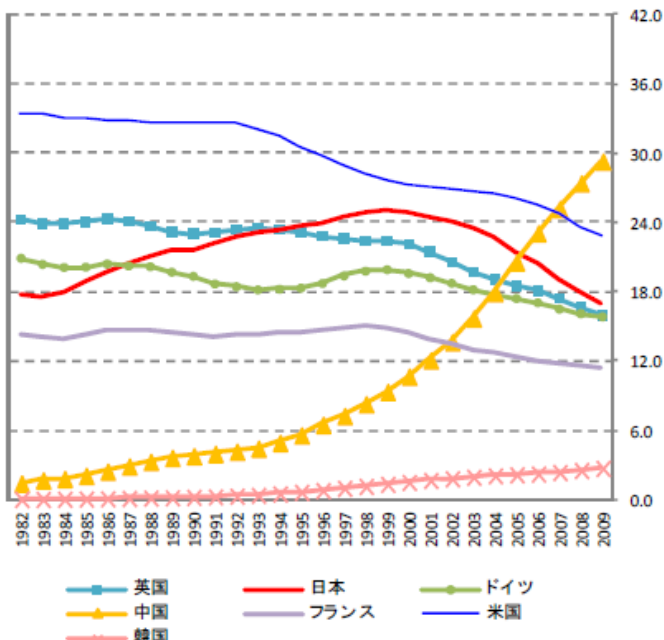
全分野での論文数(3年移動平均%) (分数カウント、米国は右軸)
