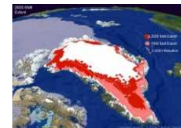
図7: グリーンランドの環境変化
