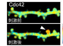
蛍光寿命二光子励起レーザー顕微鏡で測定した微小領域内での化学反応
