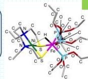
開発に成功した人工モデル触媒の構造
