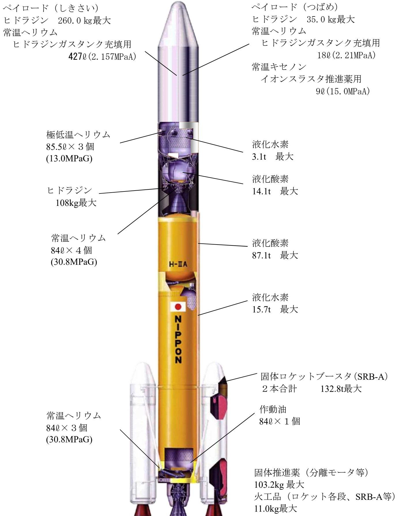
図-1 H-IIAロケット搭載用保安物概要 (火薬類、高圧ガス及び危険物)
