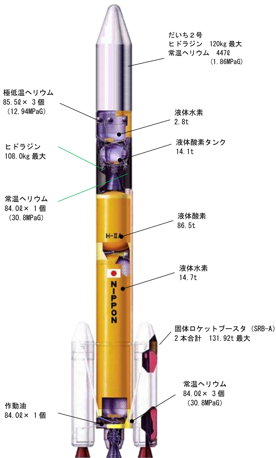
図-1 H-II A ロケット搭載用保安物概要 (火薬類、高圧ガス及び危険物)
