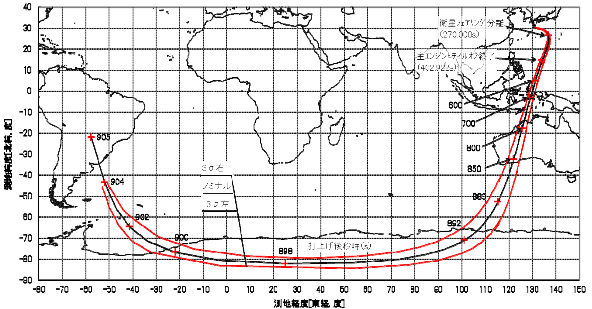
図5 (注) ロケットの落下予測点軌跡と3σ分散範囲
