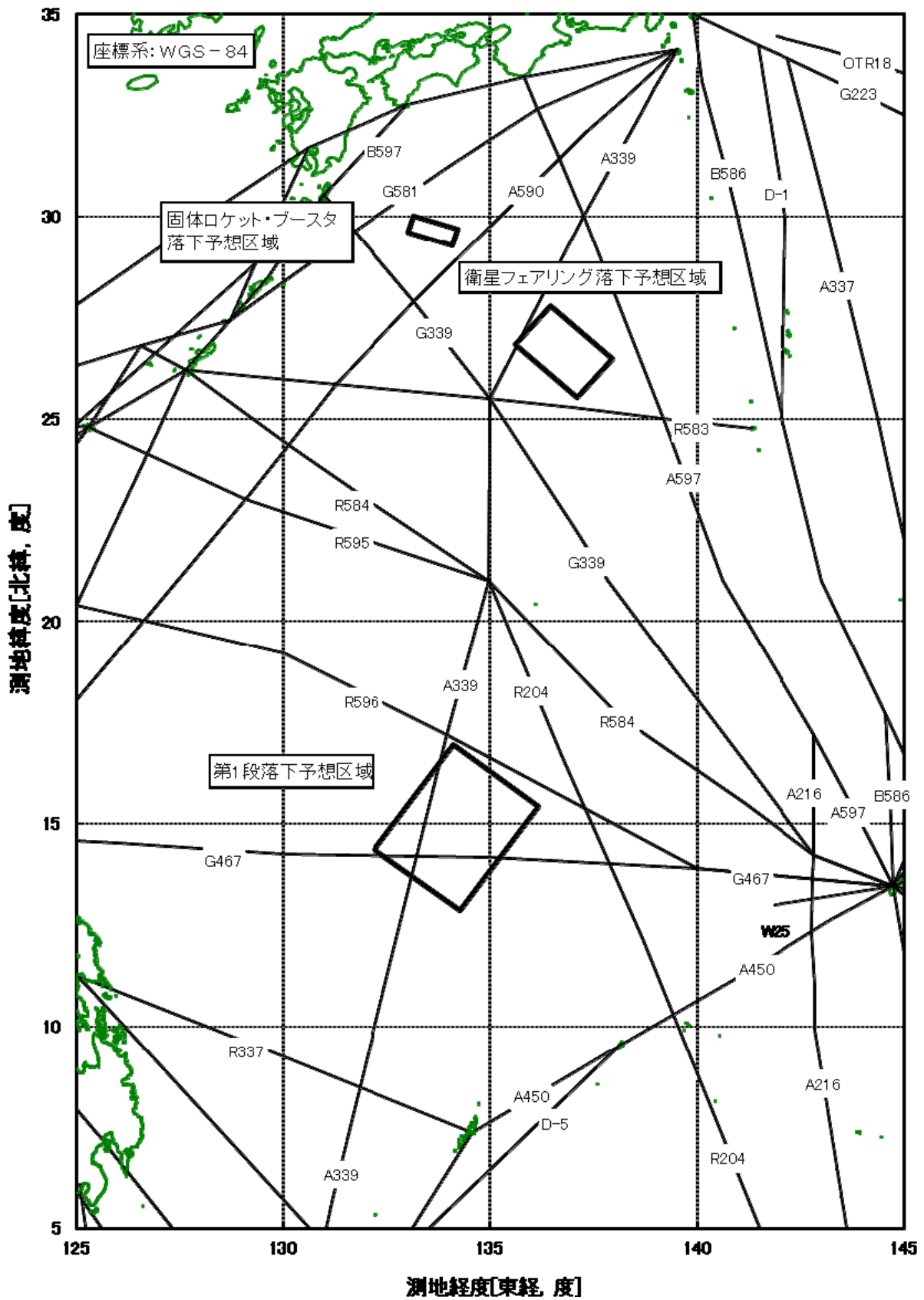
図3 落下予想区域と航空路
