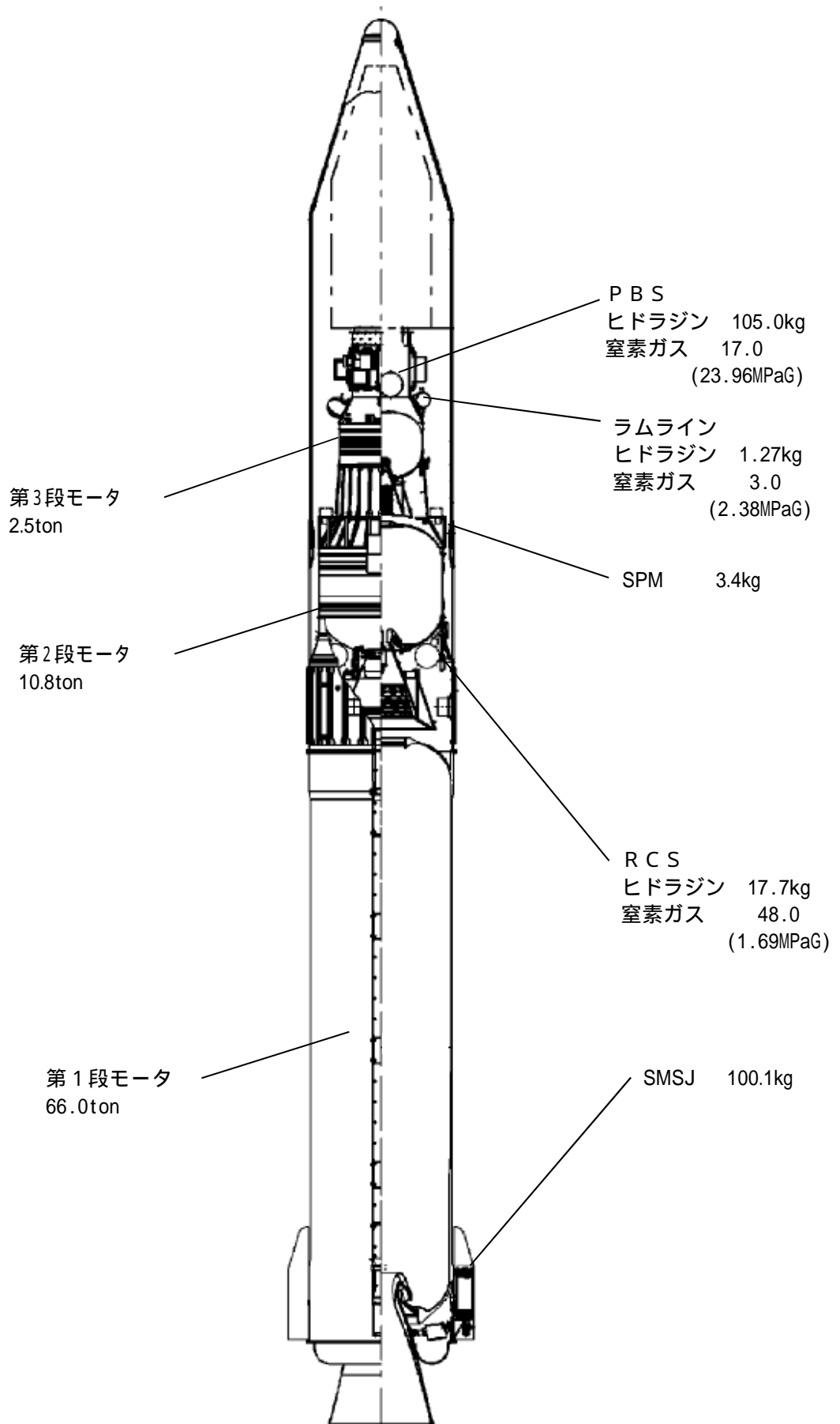
図 - 1 イブシロンロケット搭載保安物概要 (火薬類、高圧ガス、危険物)
