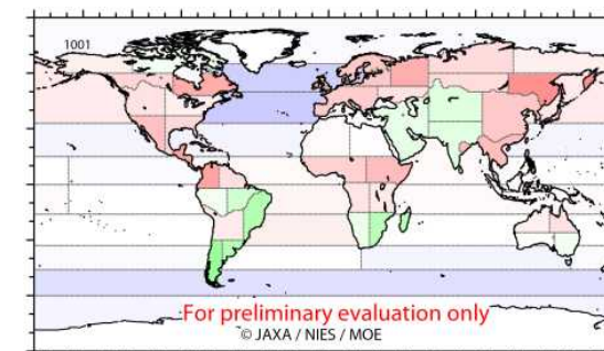
図2「いぶき」観測データを用いたCO2吸収・排出量推定結果
