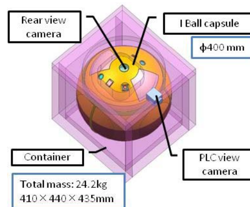
再突入データ収集装置 (2種類)
