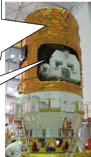
宇宙ステーション補給機(HTV) (写真はHTV2号機)
