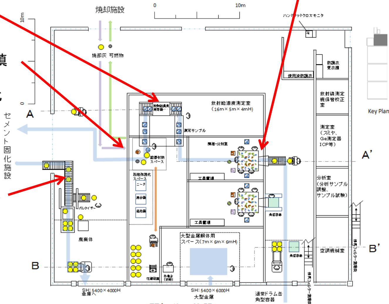
開梱分別施設1 平面図
