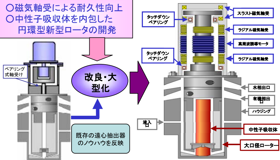
10kg/h 規模の遠心抽出器
