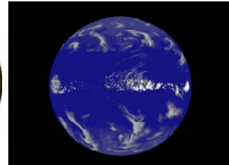
3.5kmメッシュ全球雲解像モデル による水惑星実験の雲画像
