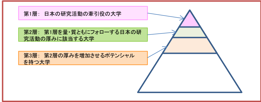
物理学分野における日本の大学の量と質の構造(2009-2013年)
