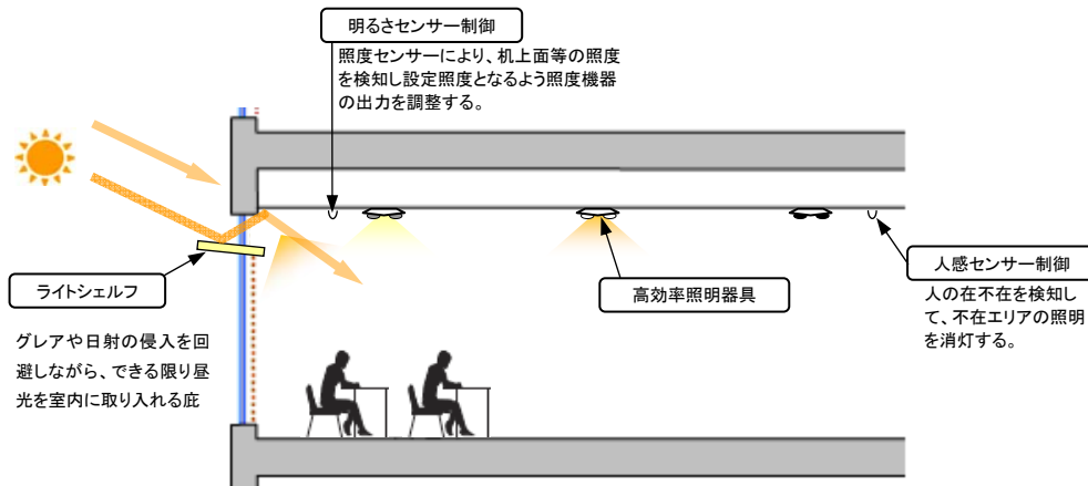
図 4.1 教室における照明エネルギー削減対策
