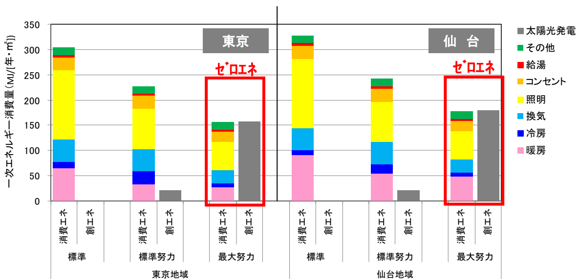
図 3.2 試算結果 (RC 造) での省エネルギー効果
