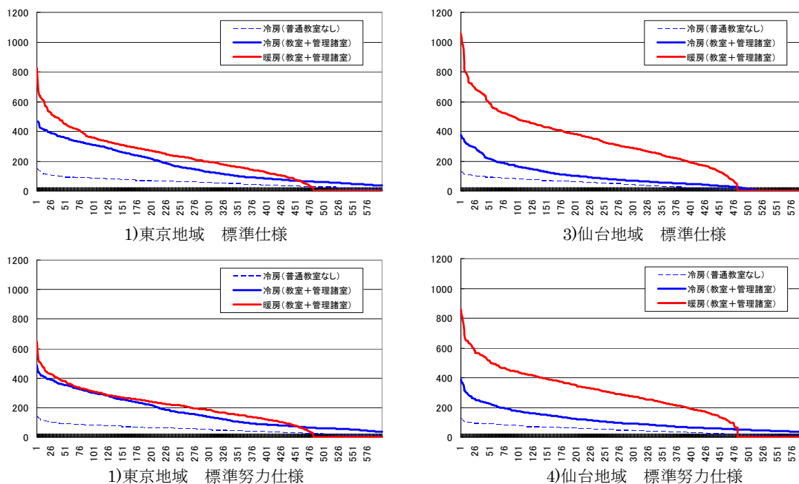
図 4.6 東京地域（温暖地）、仙台地域（寒冷地）における断熱性能の違いによる暖冷房熱負荷降順図 （縦軸：熱負荷（kW）、横軸：時間）
