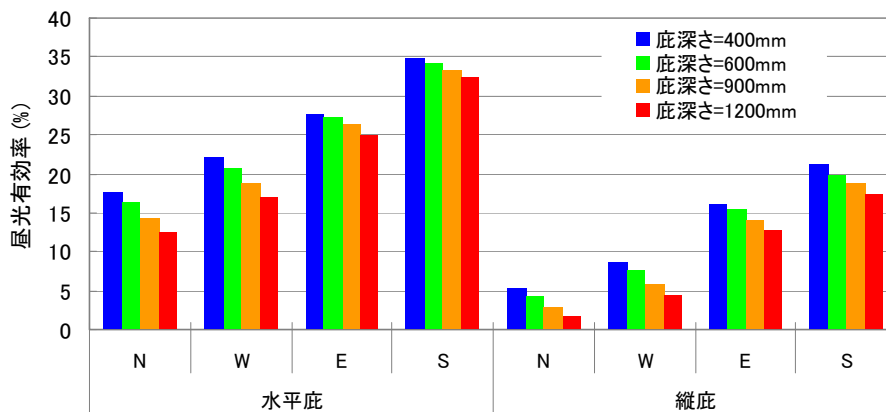
図 4.3 ライトシェルフの形状に応じた昼光有効率（人工照明消灯率）
