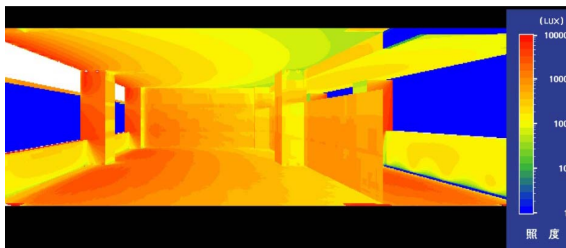
図 4.2 普通教室におけるライトシェルフによる昼光利用時の壁面照度の計算結果例
