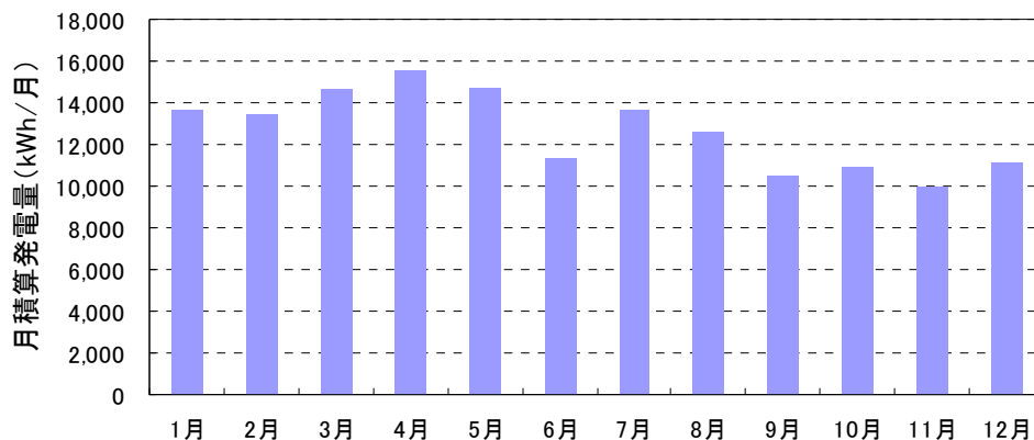
図 4.7 月毎積算発電量 (東京、最大努力ケース、定格出力 146kW)
