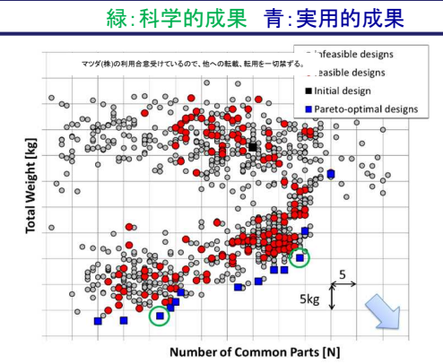
自動車車両構造設計: 従来設計よりも優れた設計を多数発見するとともに、共通部品点数最大化と重量最小化の間のトレードオフを示すことにはじめて成功
