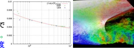
推進抵抗の比較 提供: 一般財団法人 船体まわりの渦構造 提供: 日本造船技術センター
