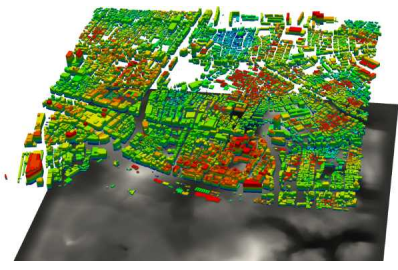
東京を対象とした地震動と建物地震応答の連成シミュレーション
