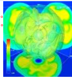
ニュートリノ加熱機構により超新星爆発が進む様子。エントロピーを表示。
