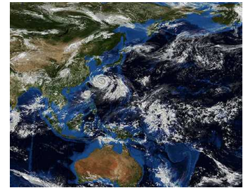
全球雲解像モデルで計算された雲と台風
