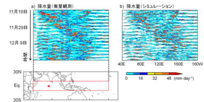
MJO予測の検証例 赤道上の降水量 経度(横軸)ー時間(縦軸)断面図 (左)観測 (右)シミュレーション
