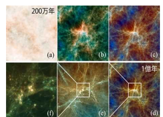
最小質量ハローの形成過程
