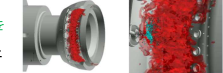
JAXA航空エンジン用アニュラ燃焼器(噴霧燃焼) 提供: 京大, JAXA
