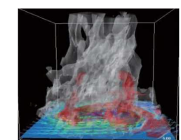
格子間隔10 mの超高解像度実験による竜巻の詳細構造
