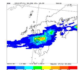
九州北部豪雨についての大雨確率予測分布図
