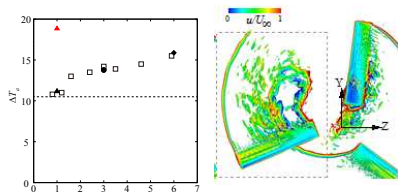
小型回転機器への適用: 実験データを再現するとともに成果②を活用した特定パラメータを利用することで大幅な性能改善が見られた。
