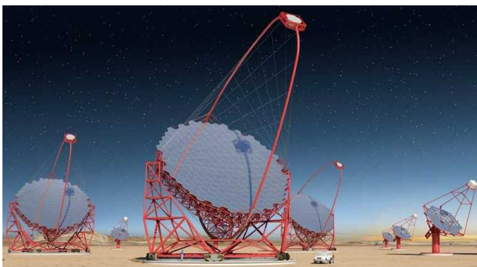
CTAイメージ。北半球には23m大口径望遠鏡4台、12m 中口径望遠鏡15台が、南半球には23m大口径望遠鏡4台、12m中口径望遠鏡25台、4m小口径望遠鏡70台が設置される。
