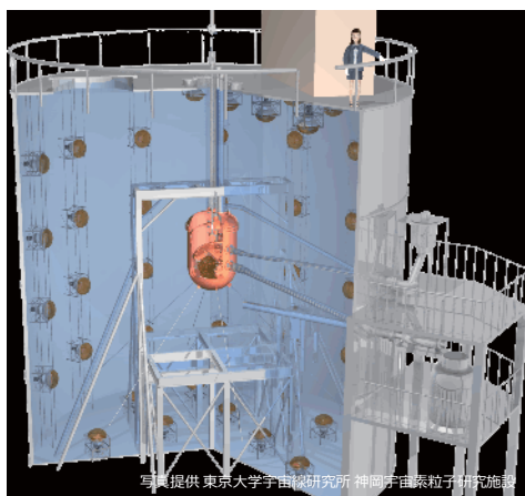
写真提供 東京大学宇宙線研究所 神岡宇宙線粒子研究施設 XMASS全体イメージ。
