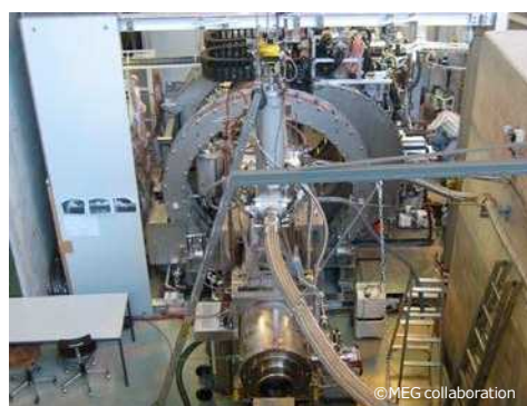
世界最大強度の陽子ビームから作った大強度ミューオンビームが通過するMEG実験ビームライン。
