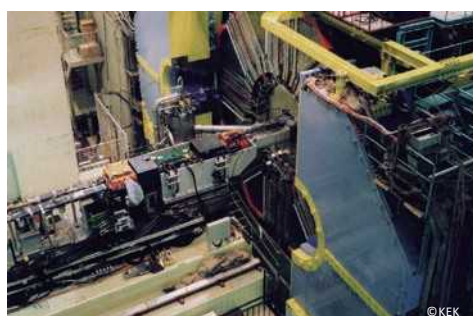
Belle検出器
