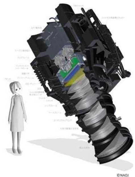
すばる望遠鏡の主焦点に設置されている、広視野CCDカメラ、Hyper Suprime-Cam (HSC)。
