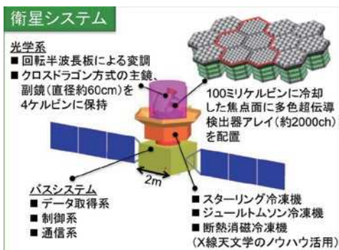
LiteBIRDイメージ
