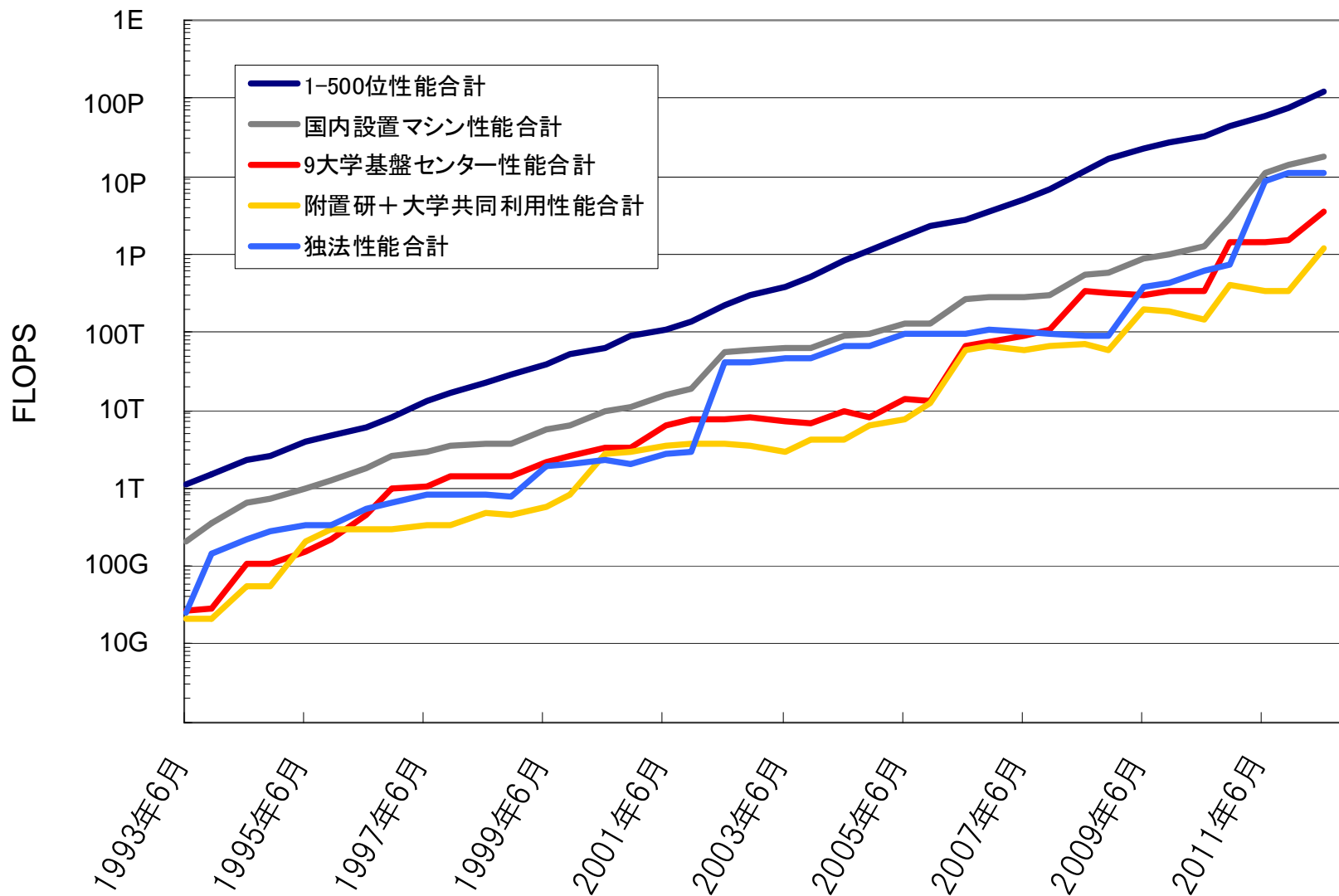
TOP500マシンと国内マシンのLINPACK性能トレンド (TOP500ランクイン分)
