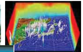
メソスケールモデル
