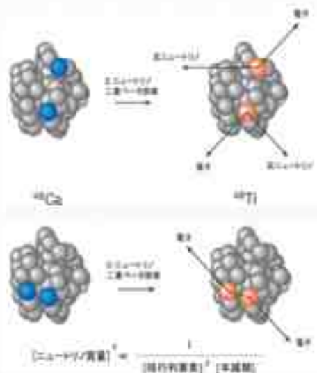
二重ベータ崩壊の模式図
