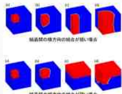
多結晶モデルの磁化反転シミュレーション (富士通プレスリリースより)
