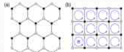
ハニカム格子および \pi フラックスを持つ正方格子の格子構造
