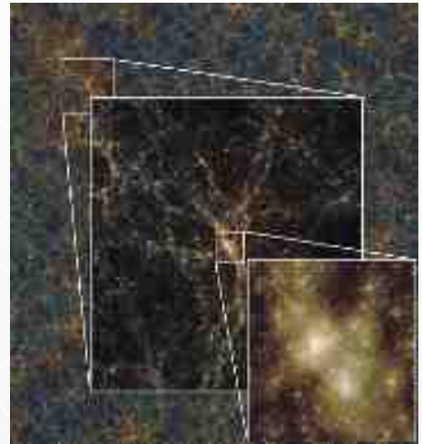
現在の宇宙でのダークマター分布 (クレジット: 国立天文台プレスリリース)
