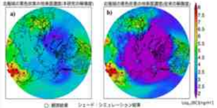
北極域の地表での黒色炭素の質量と観測との比較 (当該論文の図を用いて作成)
