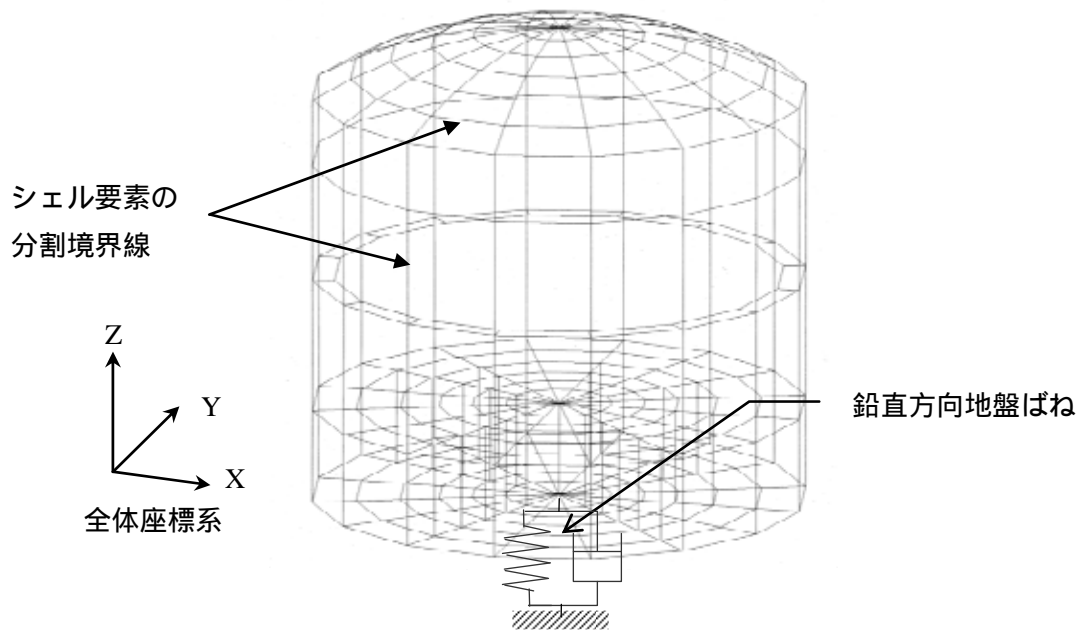
図 - 8 原子炉建屋の地震応答解析モデル（鉛直方向）
