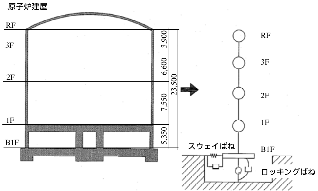
図 - 7 原子炉建屋の地震応答解析モデル（水平方向）
