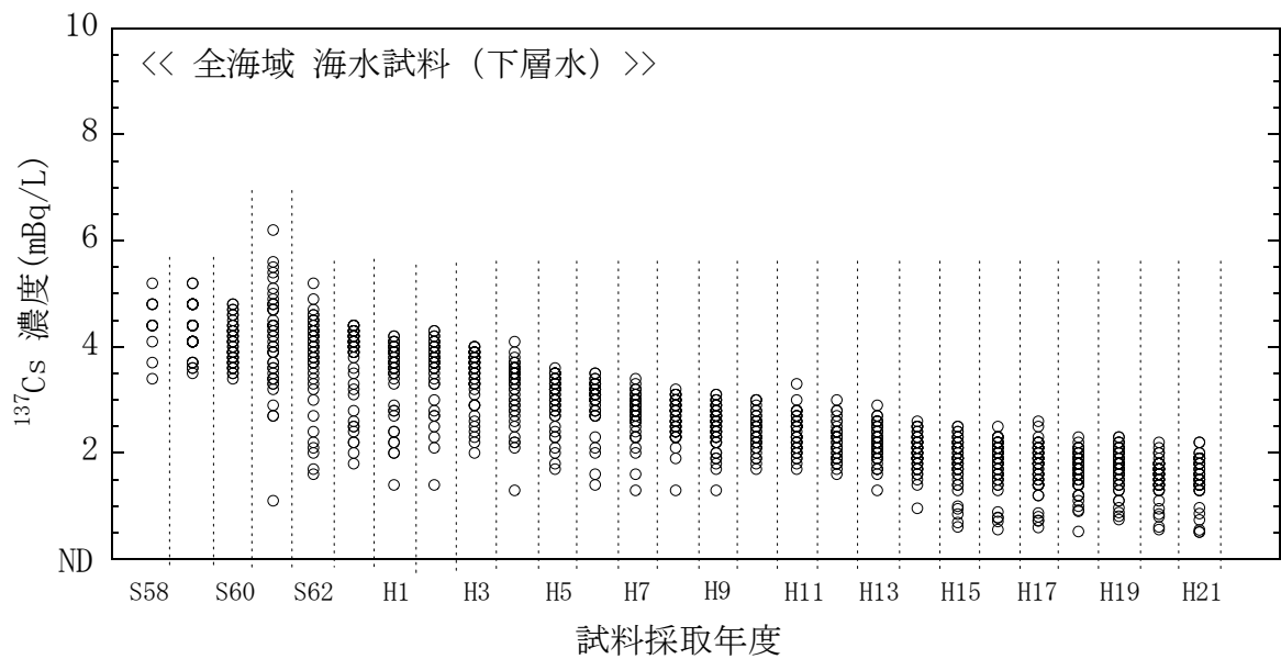
図 4(4) 海水試料のセシウム-137 濃度経年変化 (全海域・下層水)
