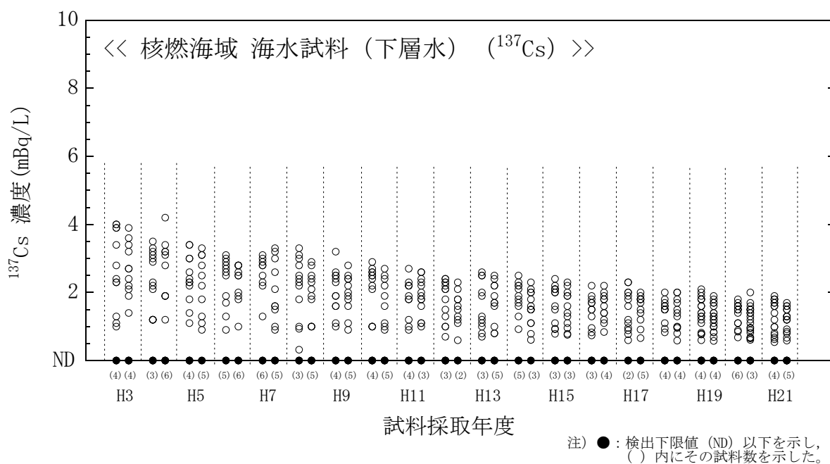
図 7(6) 海水試料のセシウム-137 濃度経年変化（核燃海域・下層水）
