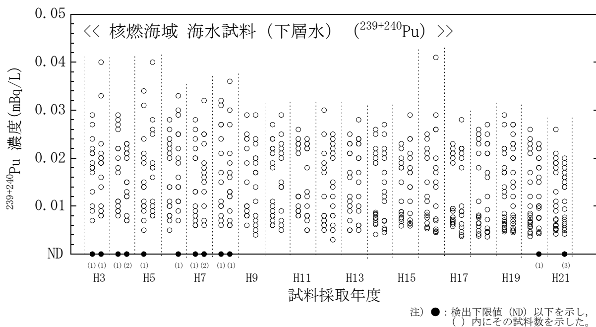
図 7(8) 海水試料のプルトニウム-239+240 濃度経年変化（核燃海域・下層水）
