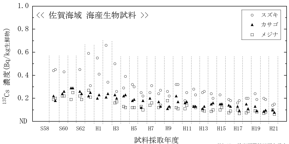
図 2(12) 海産生物試料のセシウム-137 濃度経年変化 (佐賀海域)
