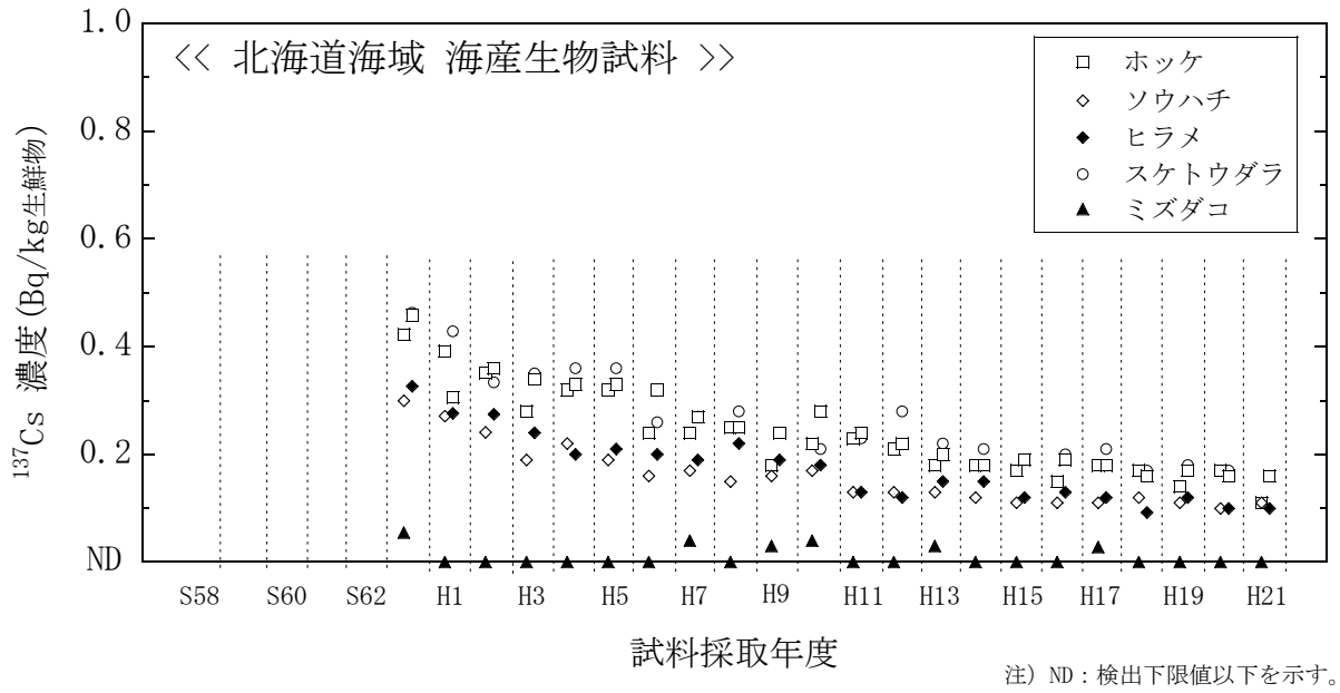
図 2(1) 海産生物試料のセシウム-137 濃度経年変化 (北海道海域)
