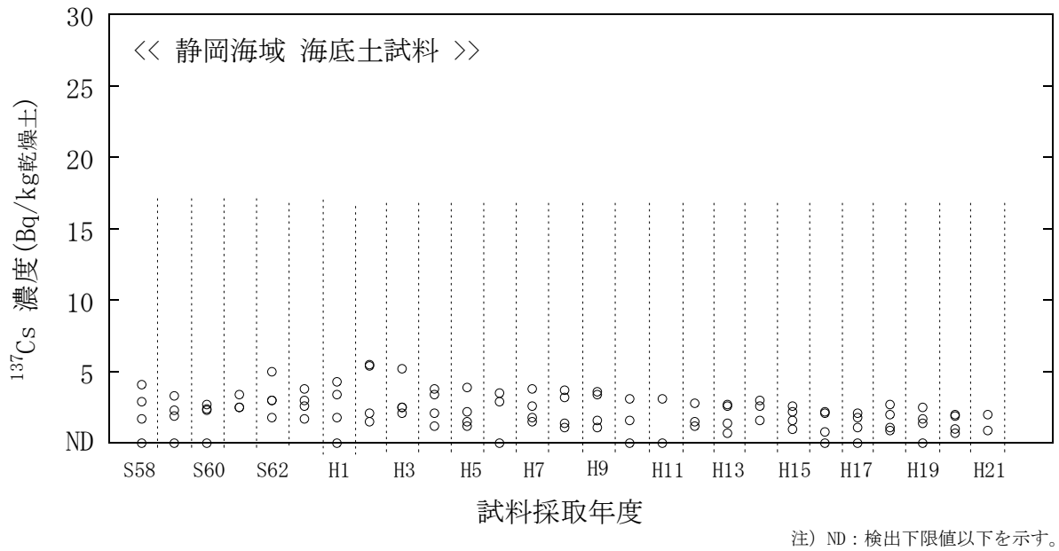
図 3(7) 海底土試料のセシウム-137 濃度経年変化 (静岡海域)
