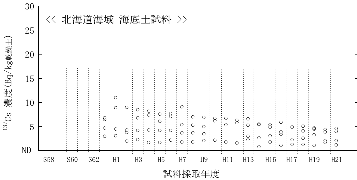
図 3(2) 海底土試料のセシウム-137 濃度経年変化 (北海道海域)
