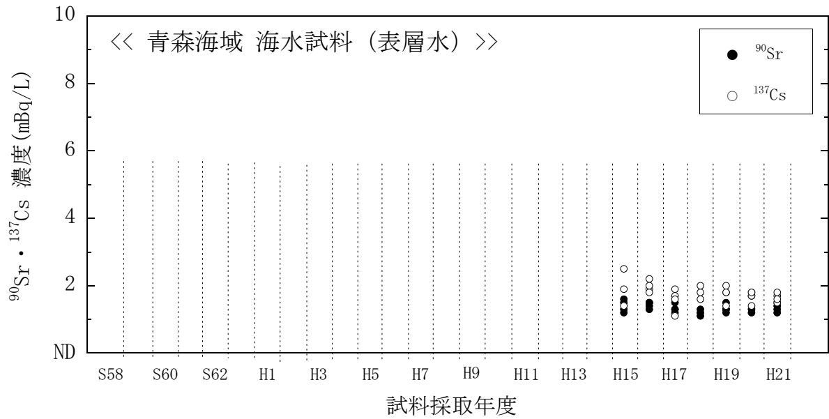
図 4(7) 海水試料のストロンチウム-90、セシウム-137 濃度の経年変化 (青森海域・表層水)
