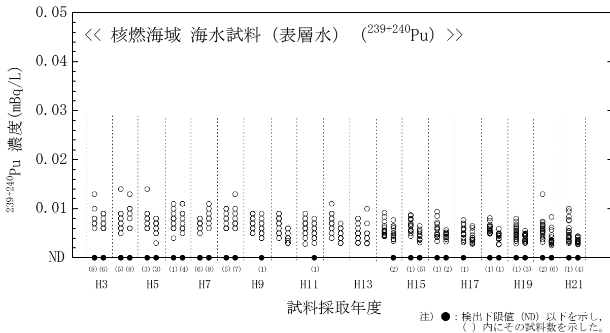
図 7(7) 海水試料のプルトニウム-239+240 濃度経年変化（核燃海域・表層水）
