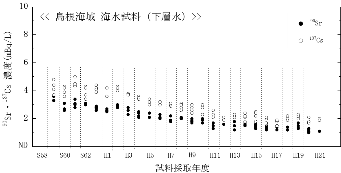
図 4(24) 海水試料のストロンチウム-90、セシウム-137 濃度の経年変化 (島根海域・下層水)
