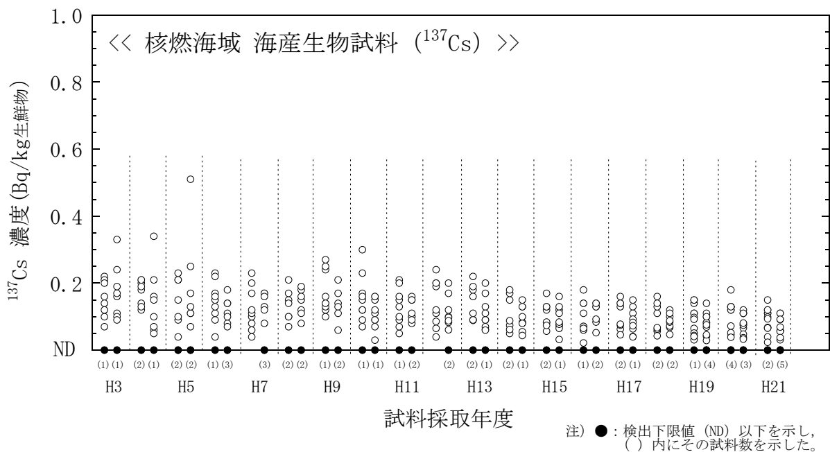
図 5(2) 海産生物試料のセシウム-137 濃度経年変化 (核燃海域)
