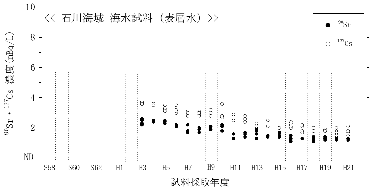
図 4(19) 海水試料のストロンチウム-90、セシウム-137 濃度の経年変化 (石川海域・表層水)
