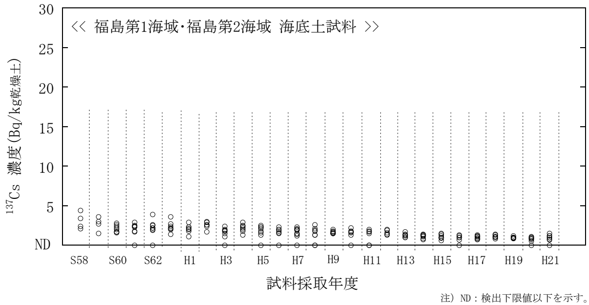
図 3(5) 海底土試料のセシウム-137 濃度経年変化 (福島第1海域・福島第2海域)
