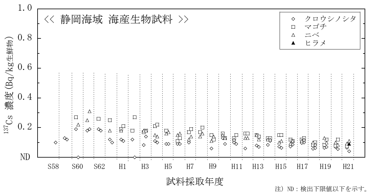
図 2(6) 海産生物試料のセシウム-137 濃度経年変化 (静岡海域)
