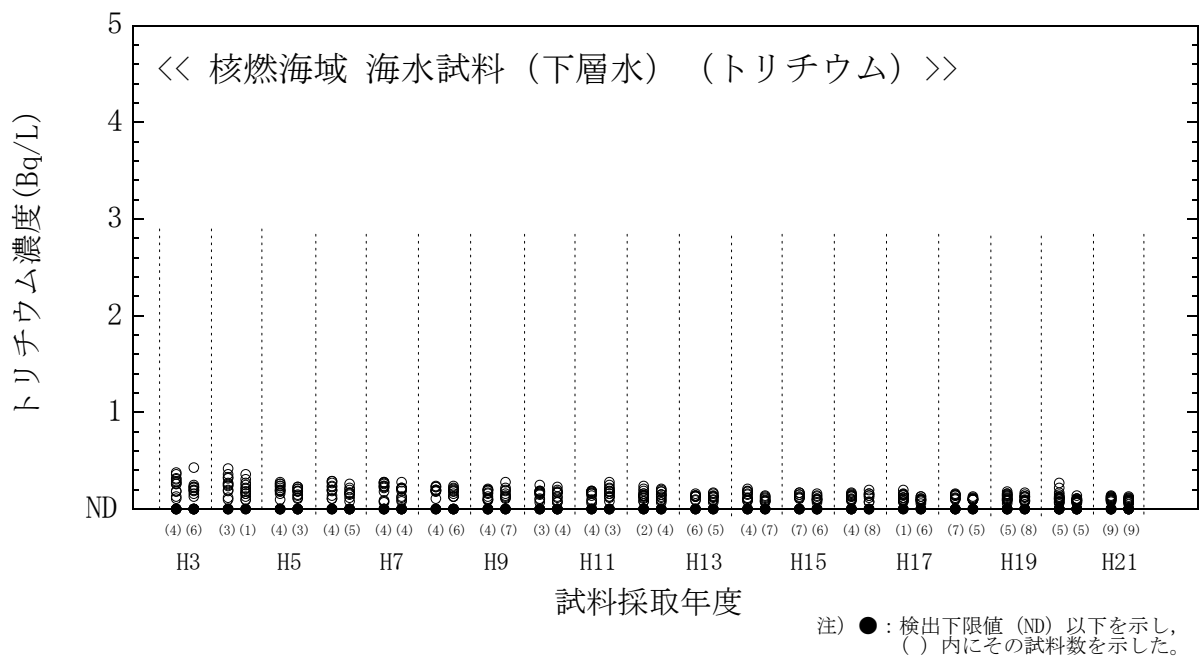
図 7(2) 海水試料のトリチウム濃度経年変化（核燃海域・下層水）
