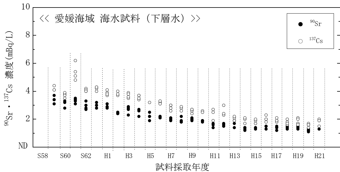
図 4(26) 海水試料のストロンチウム-90、セシウム-137 濃度の経年変化 (愛媛海域・下層水)
