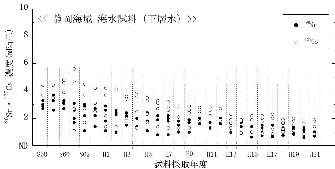
図 4(16) 海水試料のストロンチウム-90、セシウム-137 濃度の経年変化 (静岡海域・下層水)
