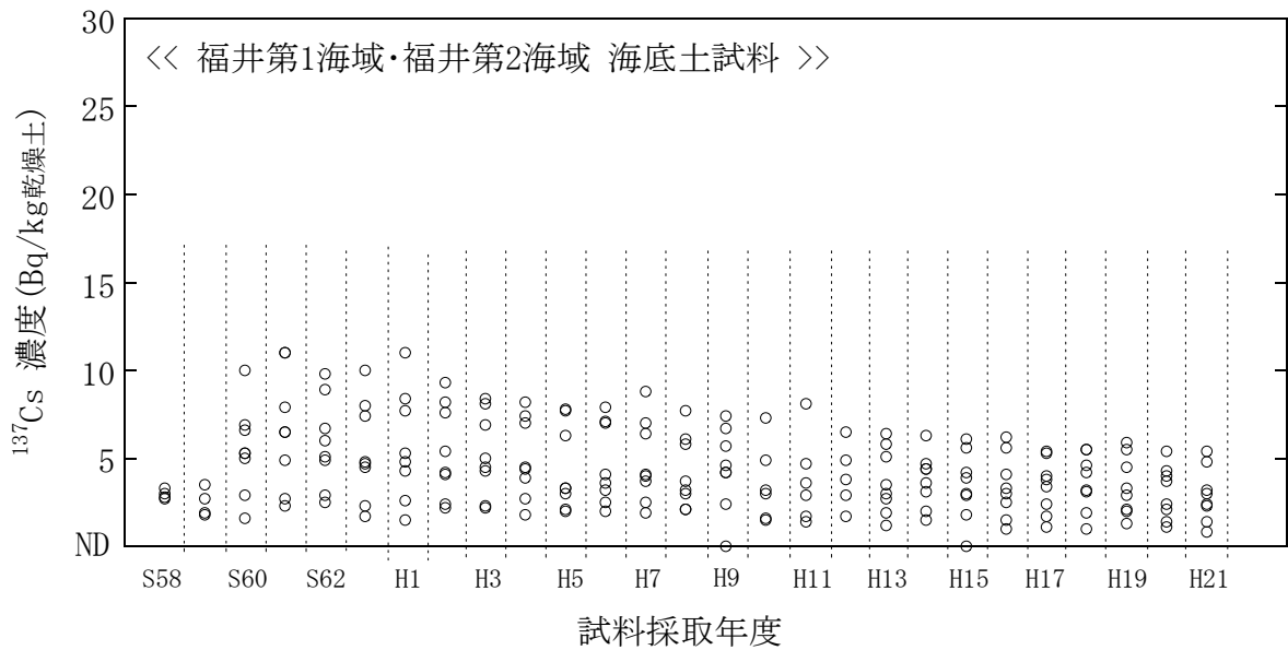
図 3(10) 海底土試料のセシウム-137 濃度経年変化 (福井第1海域・福井第2海域)
