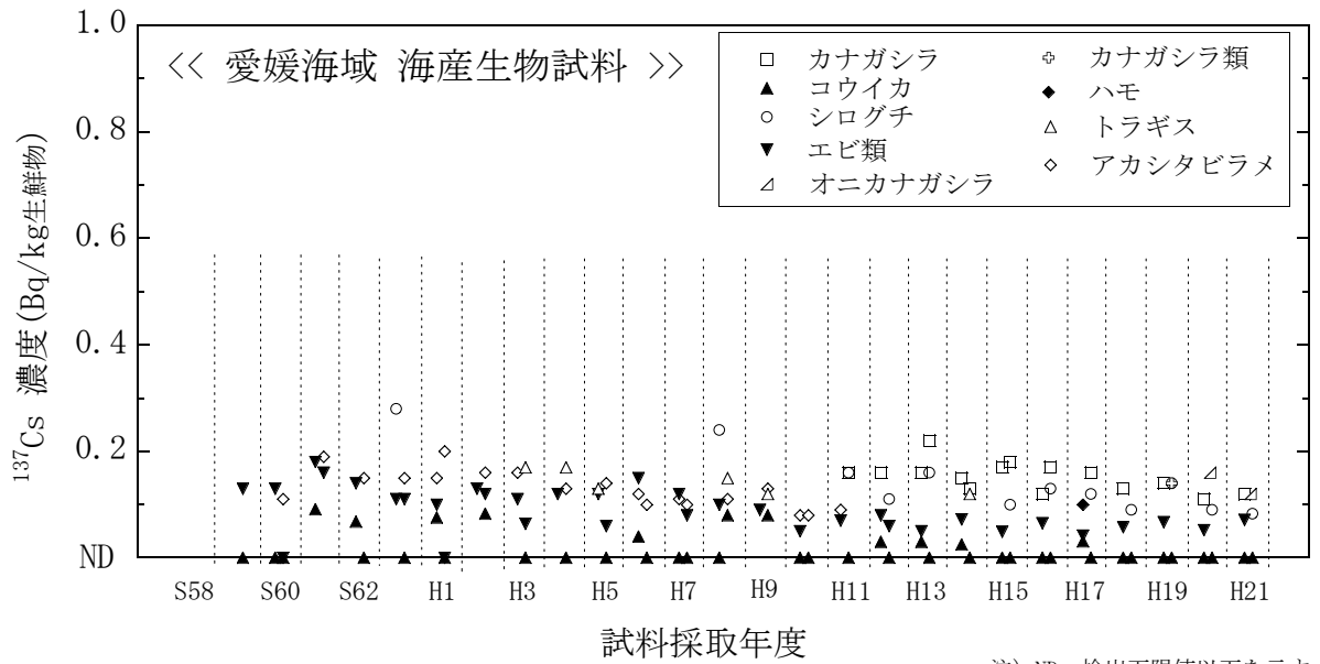
図 2(11) 海産生物試料のセシウム-137 濃度経年変化 (愛媛海域)
