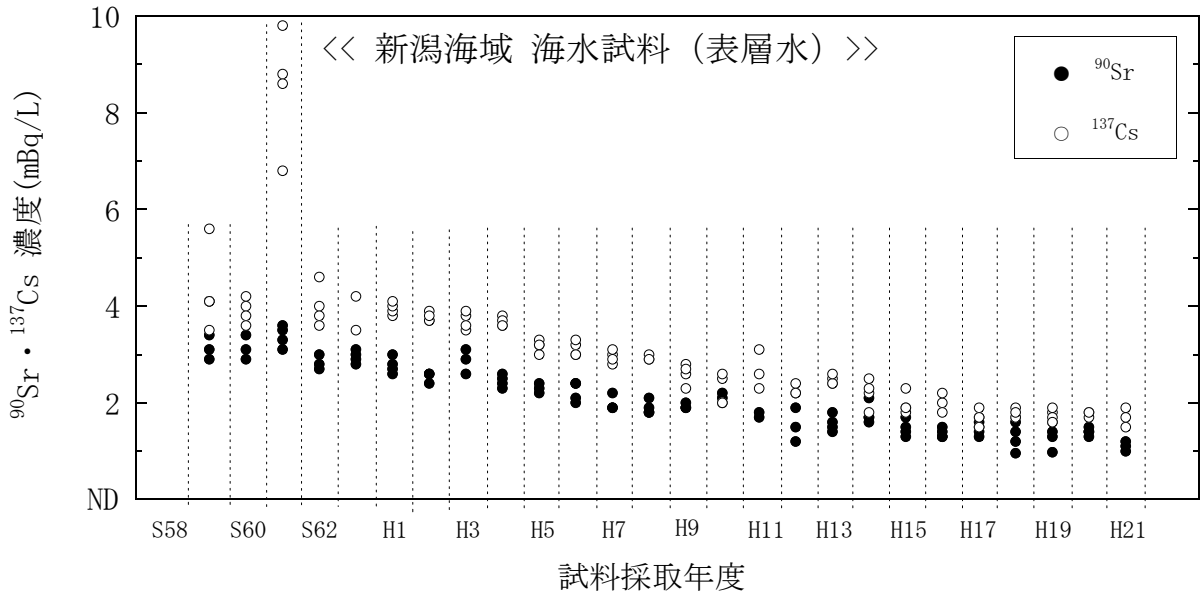
図 4(17) 海水試料のストロンチウム-90、セシウム-137 濃度の経年変化 (新潟海域・表層水)
