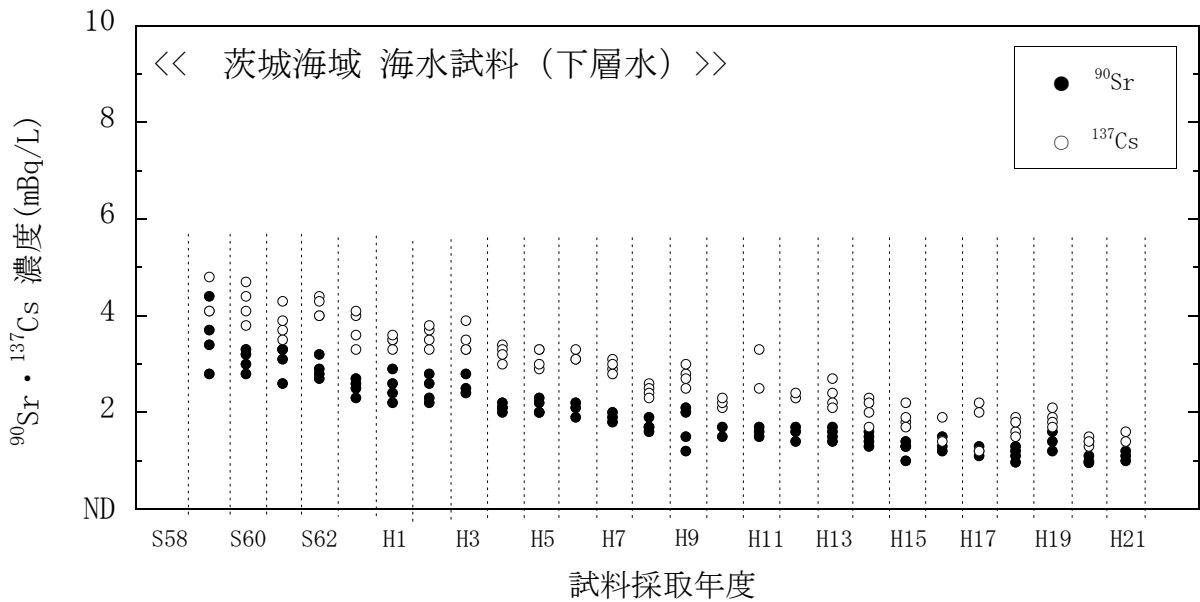
図 4(14) 海水試料のストロンチウム-90、セシウム-137 濃度の経年変化 (茨城海域・下層水)
