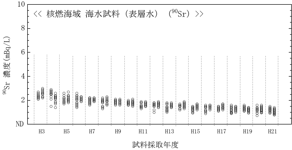
図 7(3) 海水試料のストロンチウム-90 濃度経年変化（核燃海域・表層水）
