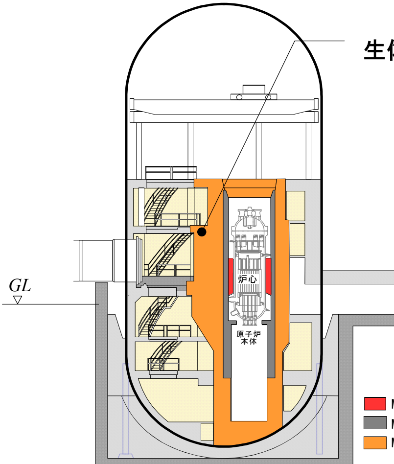
JPDR, 90MWth BWR
