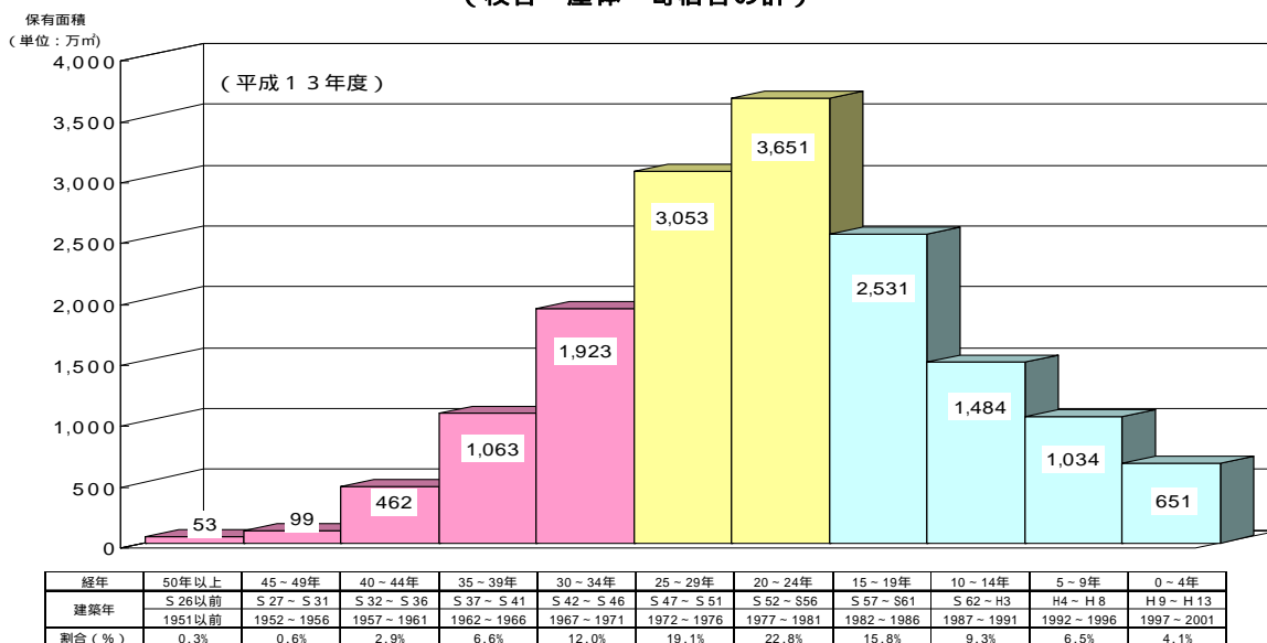
公立小中学校非木造建物の経年別保有面積 < 全国 > (校舎・屋体・寄宿舎の計)
